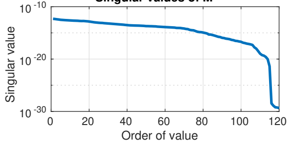
(d) Singular values of M
