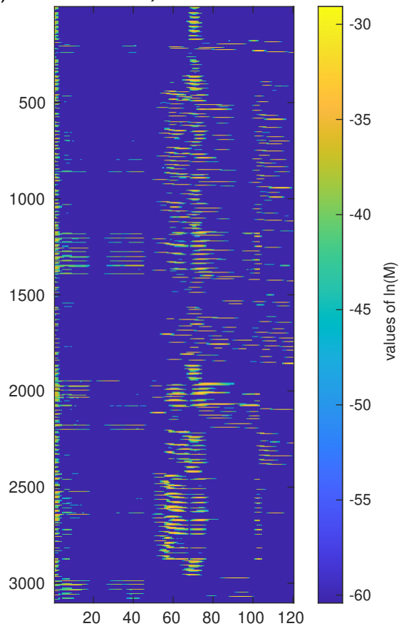
(d) Singular values of M
