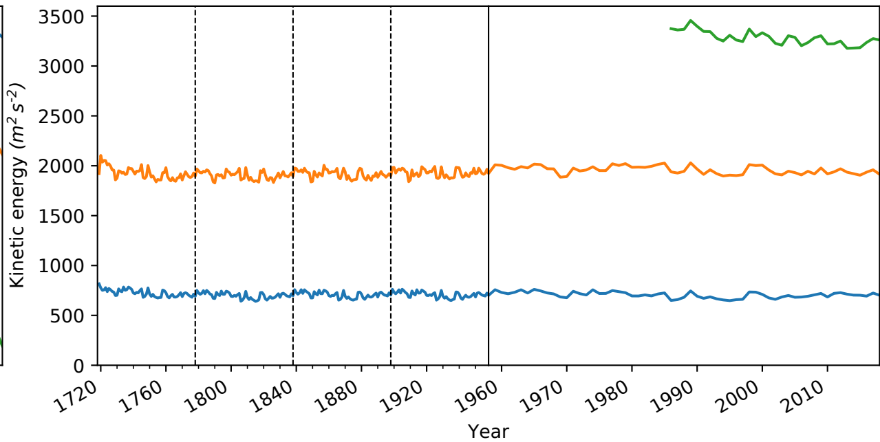
(d) Global average kinetic energy
