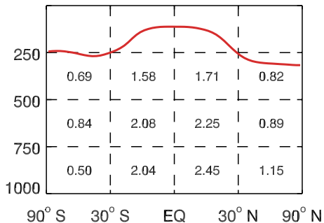
(d) BCC-GEOS-Chem
