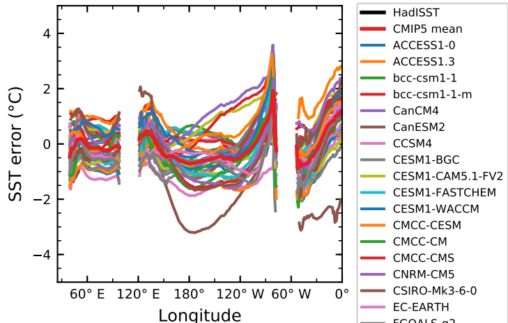
(d) Equatorial SST error CMIP5
