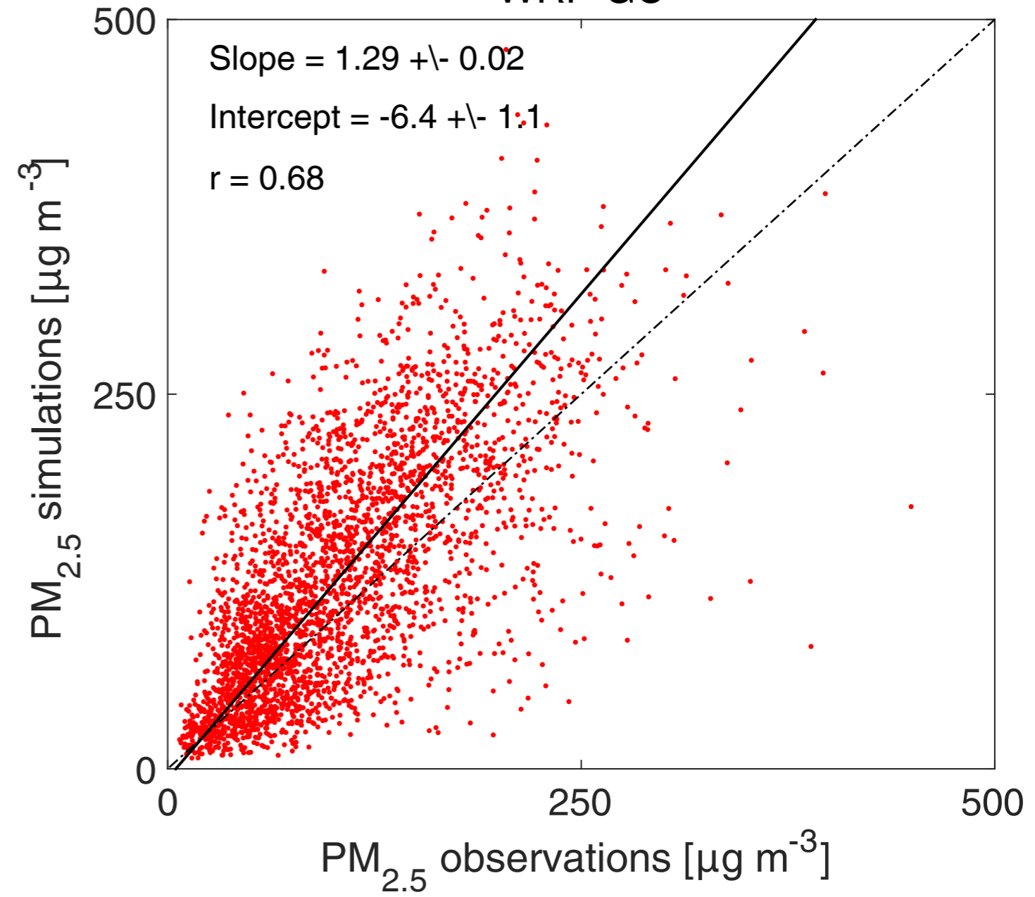
WRF-GC
