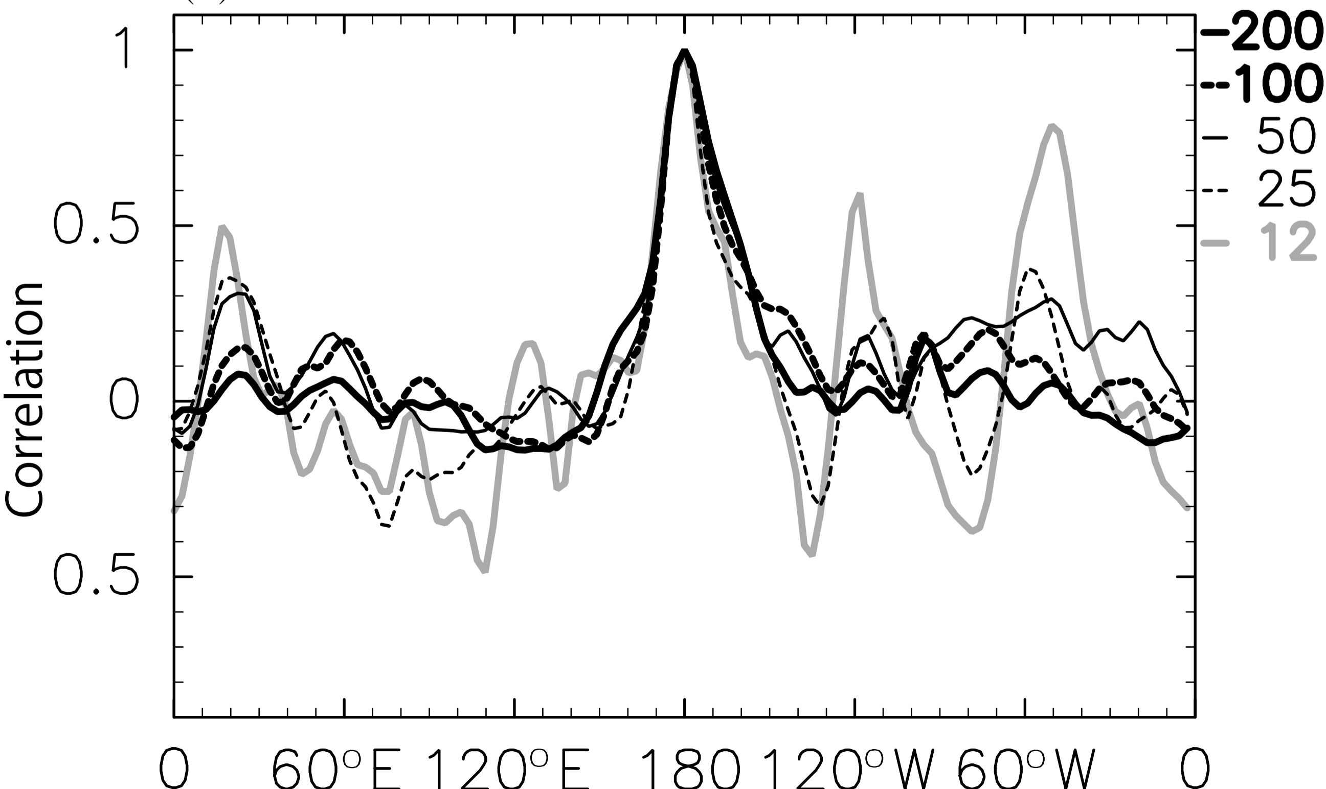
(b) 0.01 hPa
