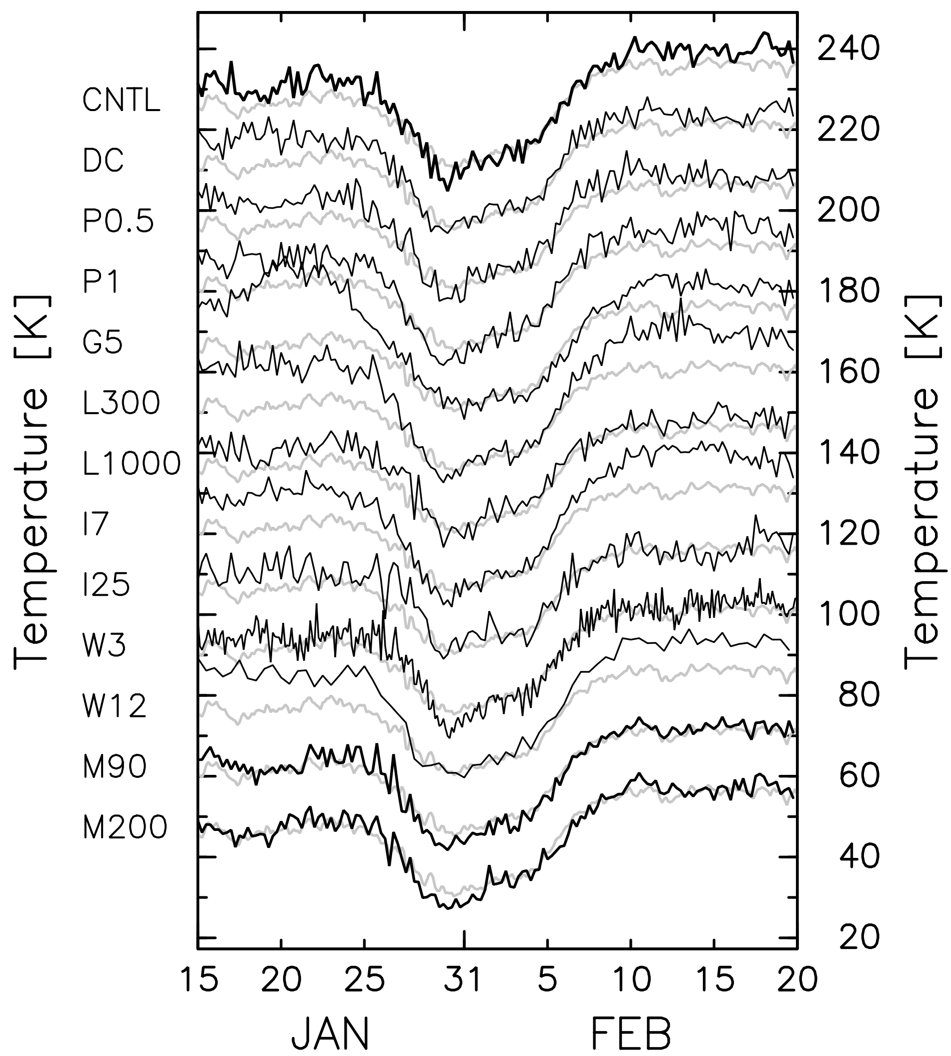
(d) T 0.1 hPa 70° N
