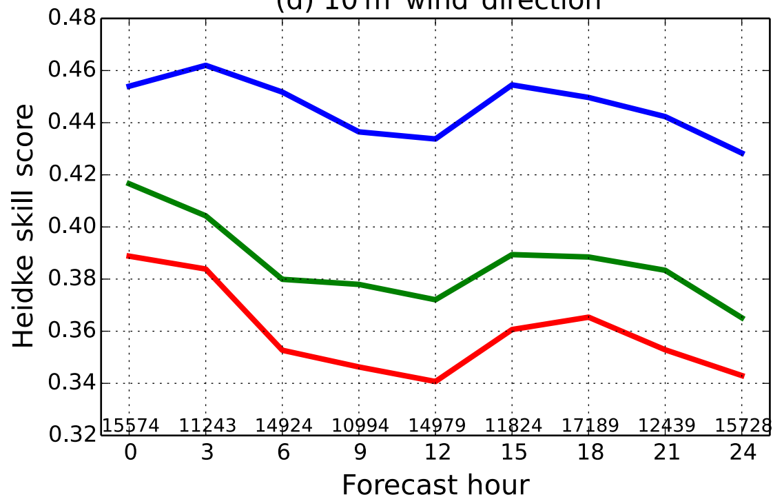
(d) 10 m wind direction
