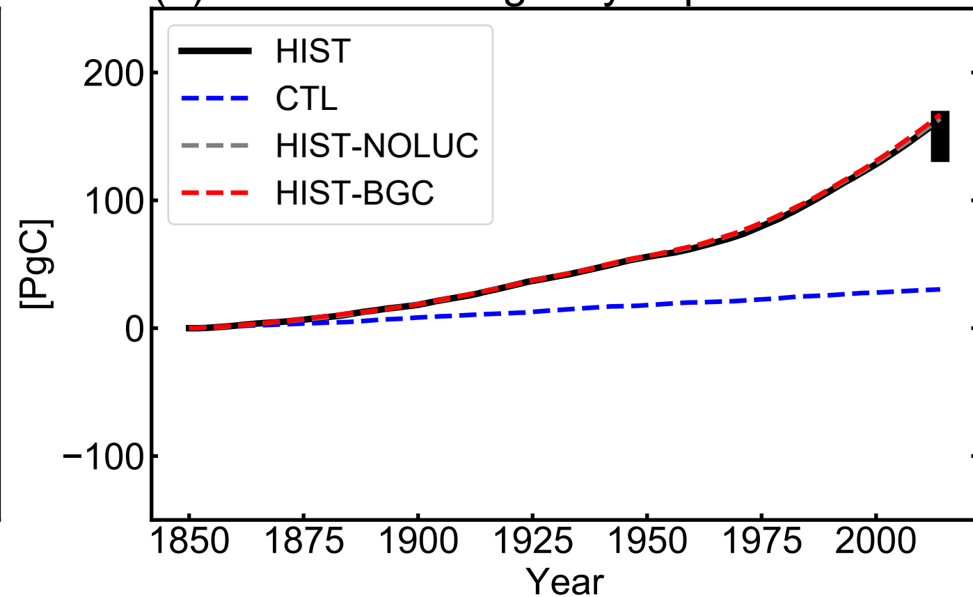
(d) Ocean C change: by responses
