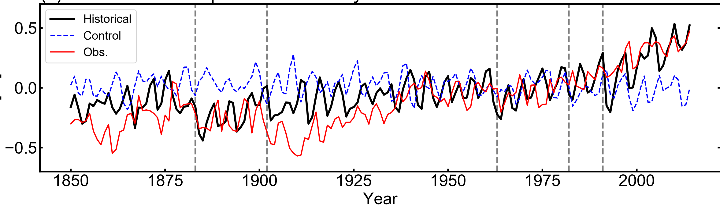
(d) Ocean temperature at 0–700 m
