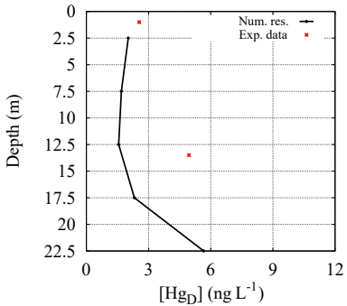
(d) Hg D concentration (station 15)
