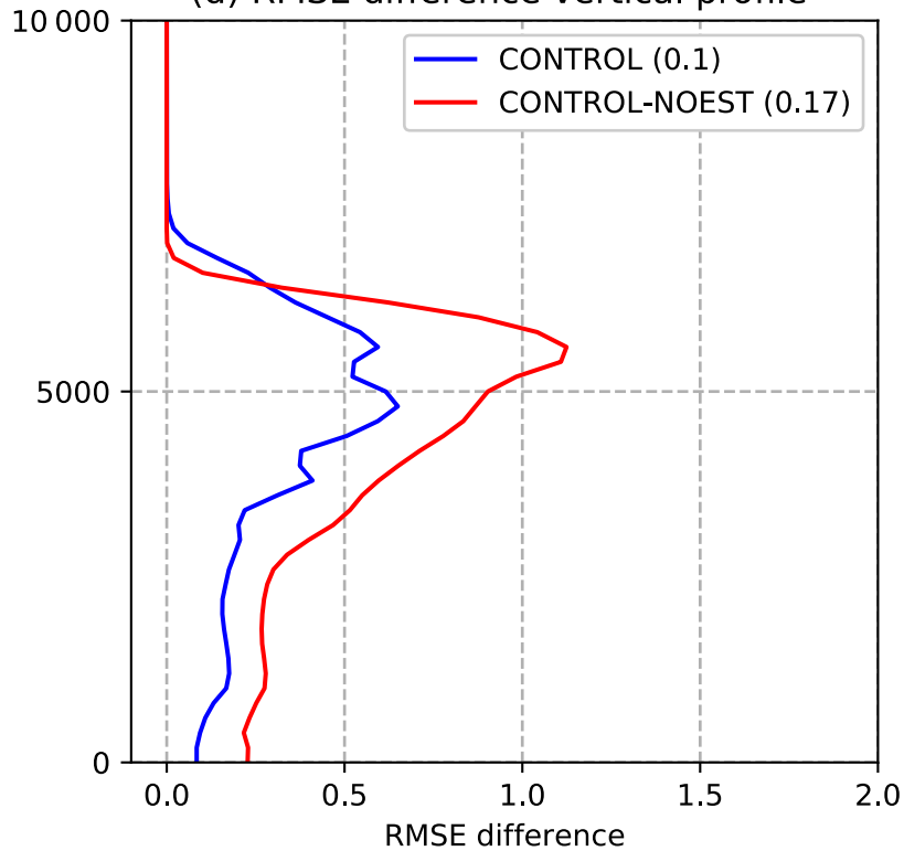
(d) RMSE difference vertical profile
