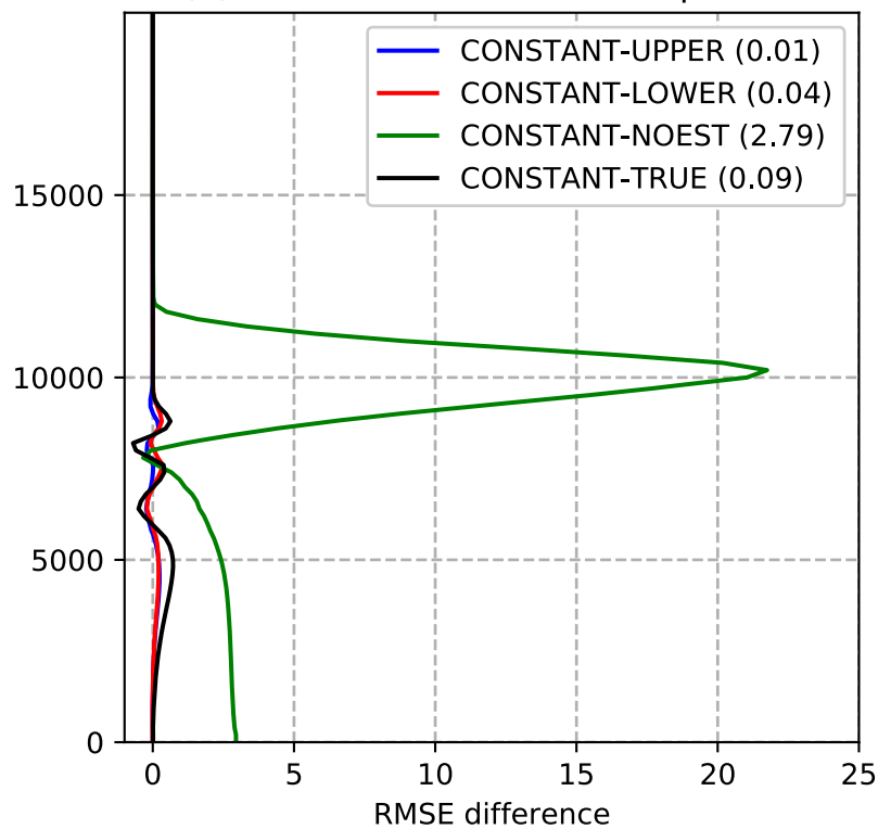
(d) RMSE difference vertical profile
