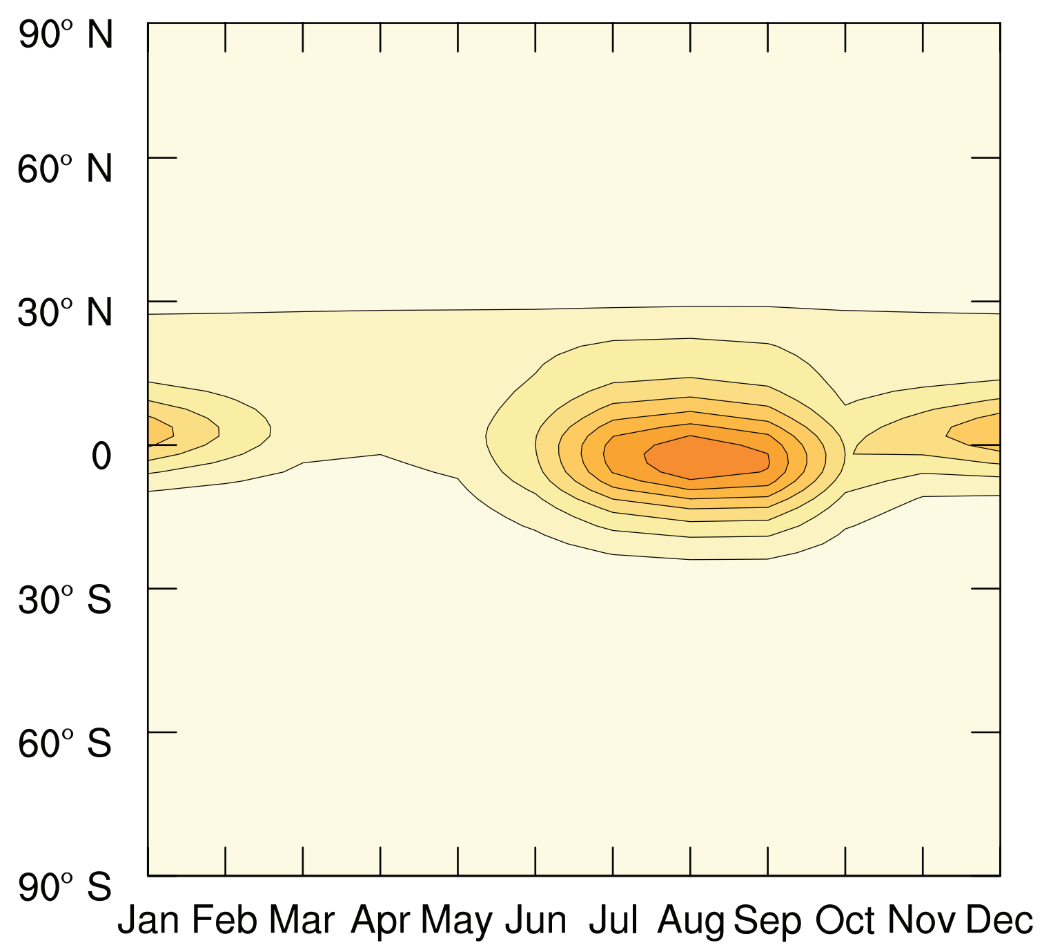
SSP3-LowNTCF
