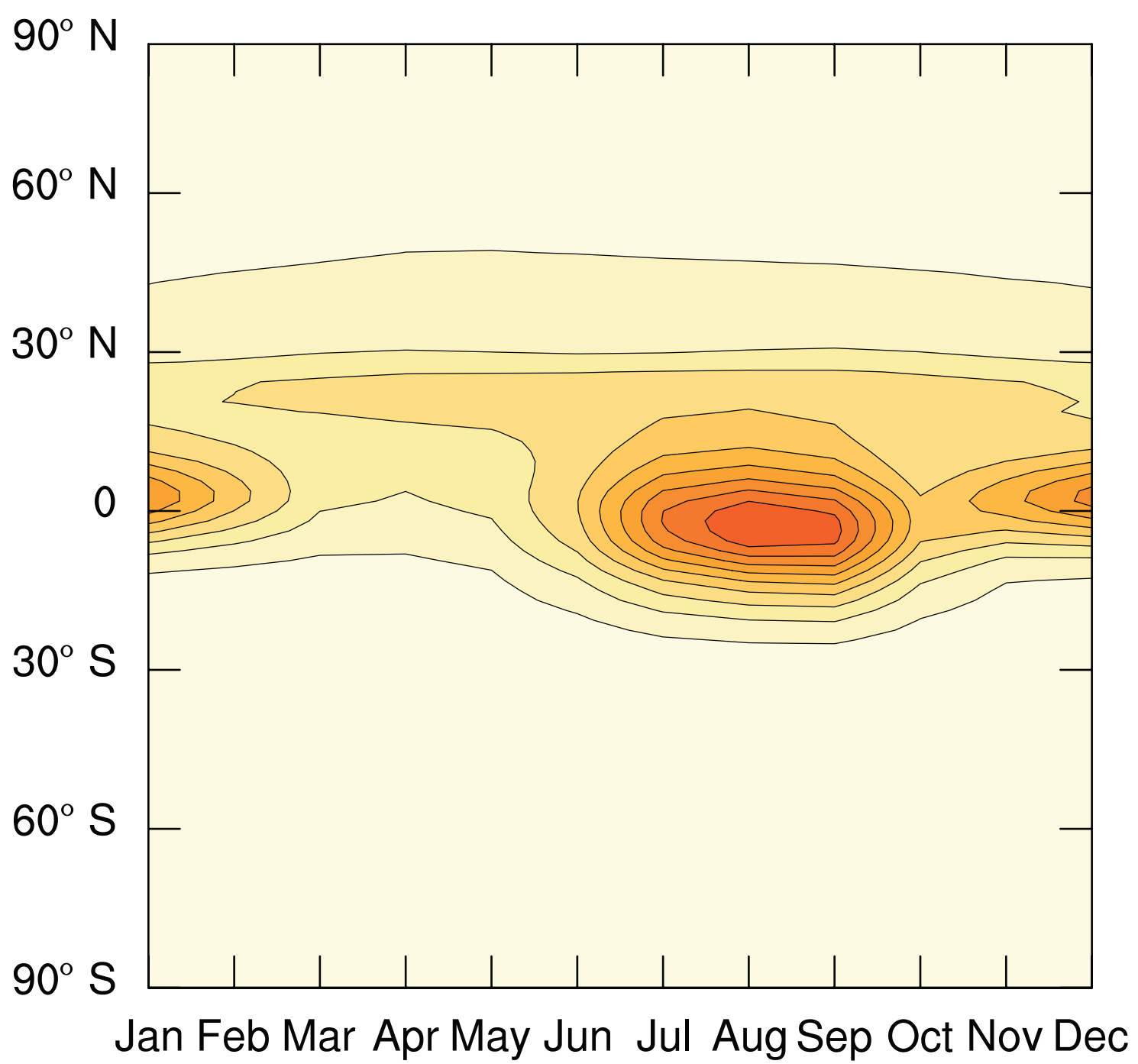
SSP3-LowNTCF
