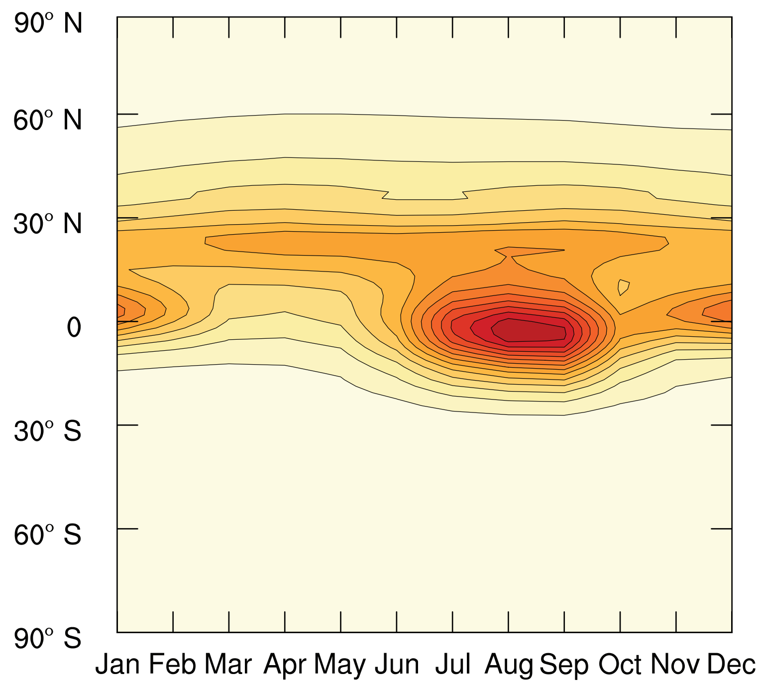
SSP3-70
