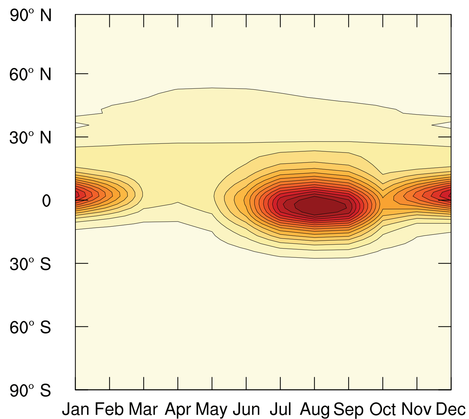
SSP5-85
