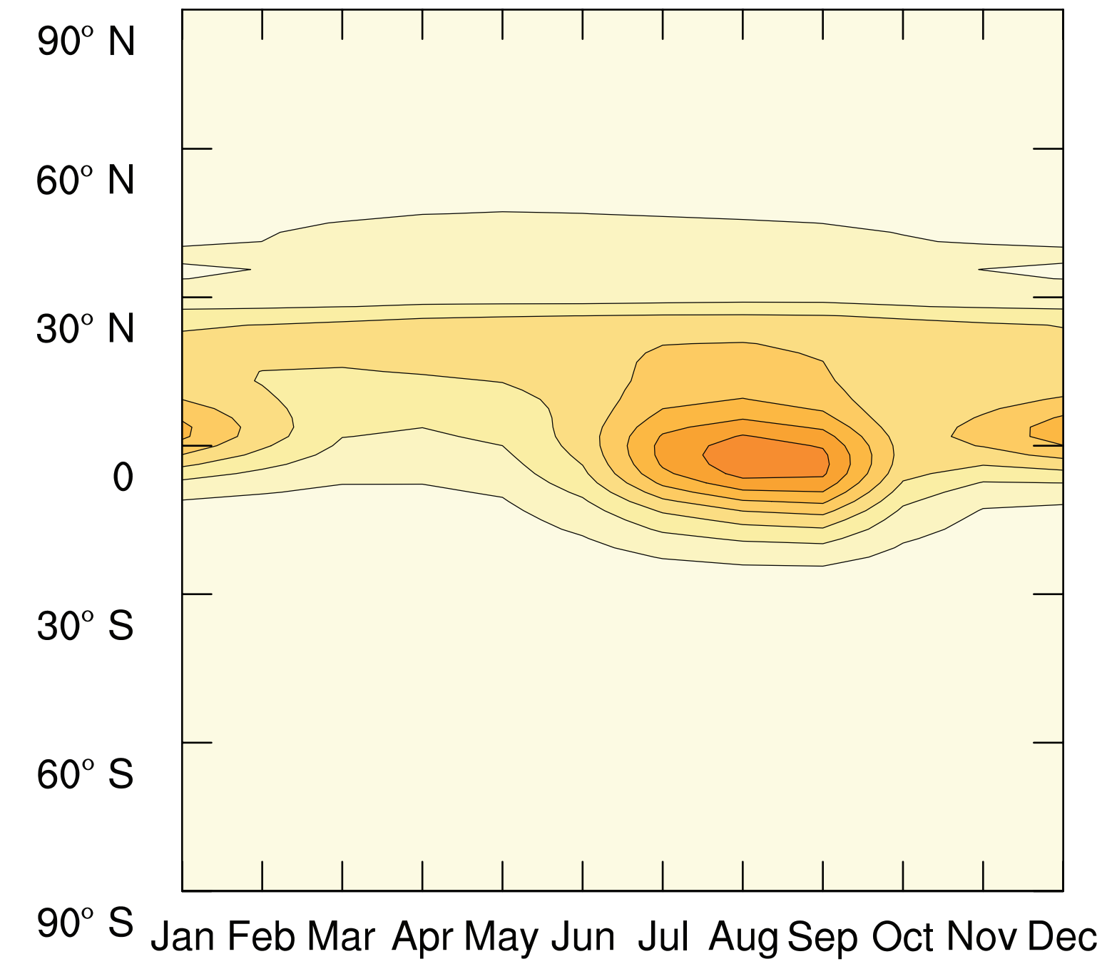
SSP4-34
