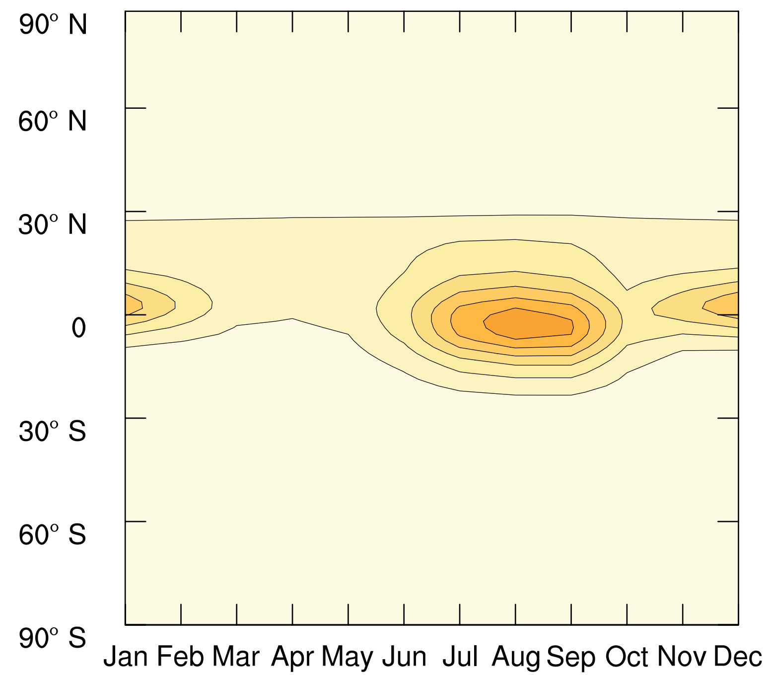
SSP3-70
