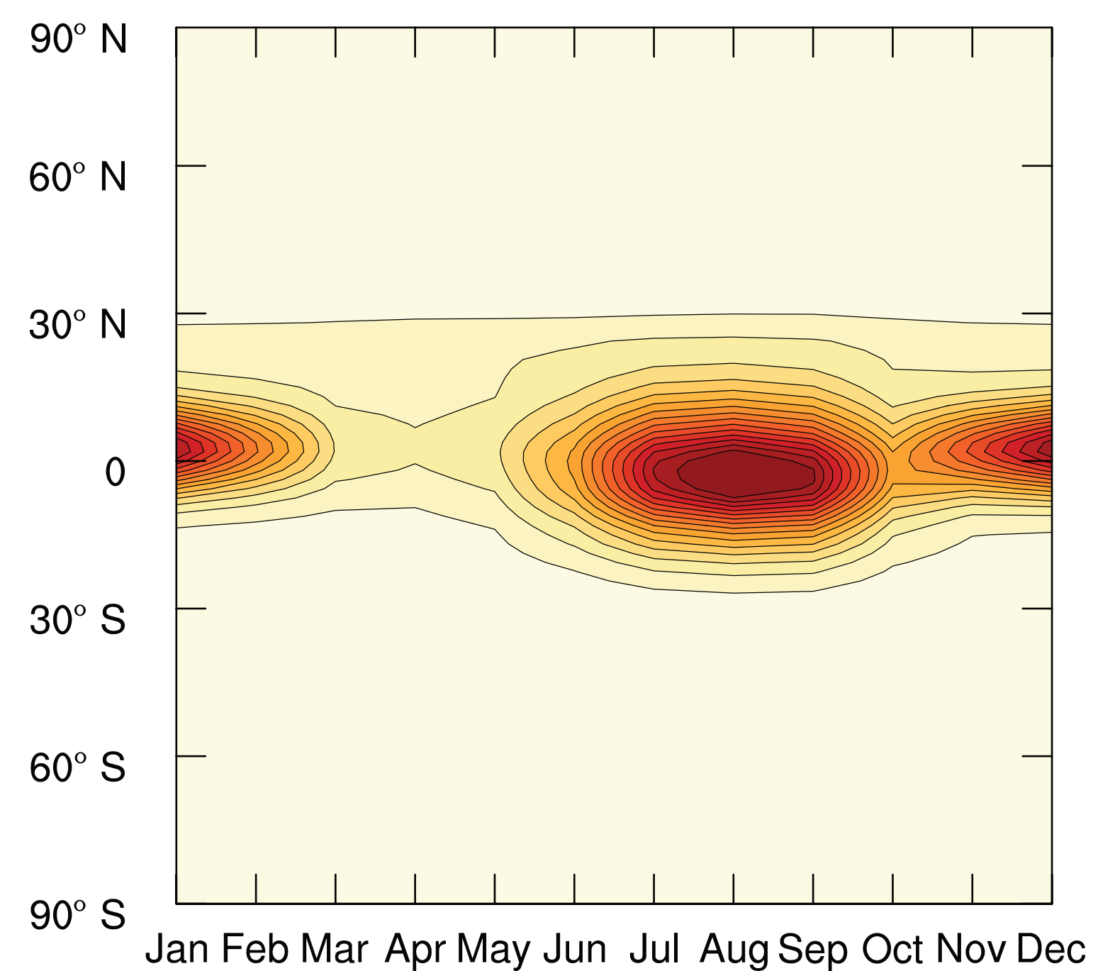
SSP4-34
