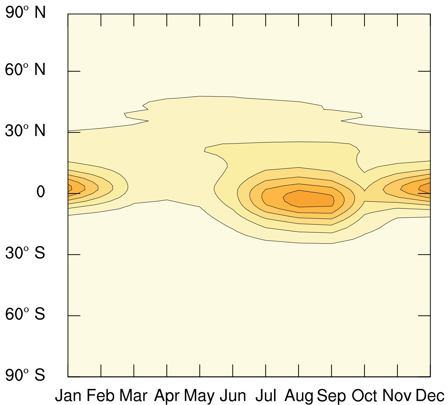
SSP5-34-OS
