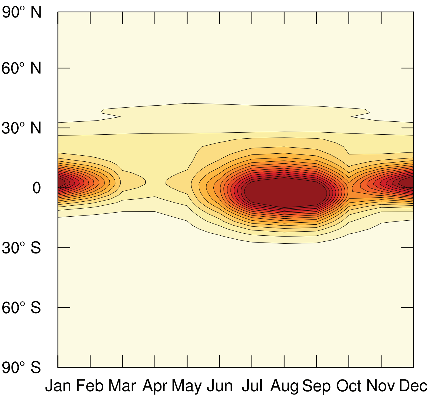
SSP4-60
