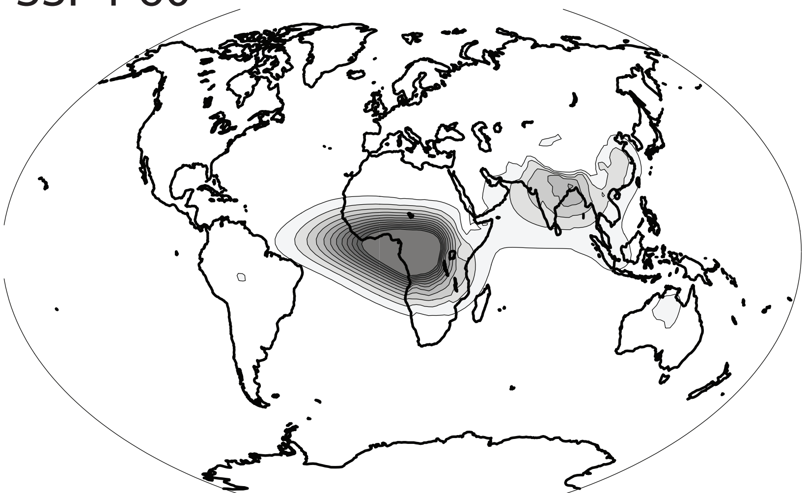
SSP4-60
