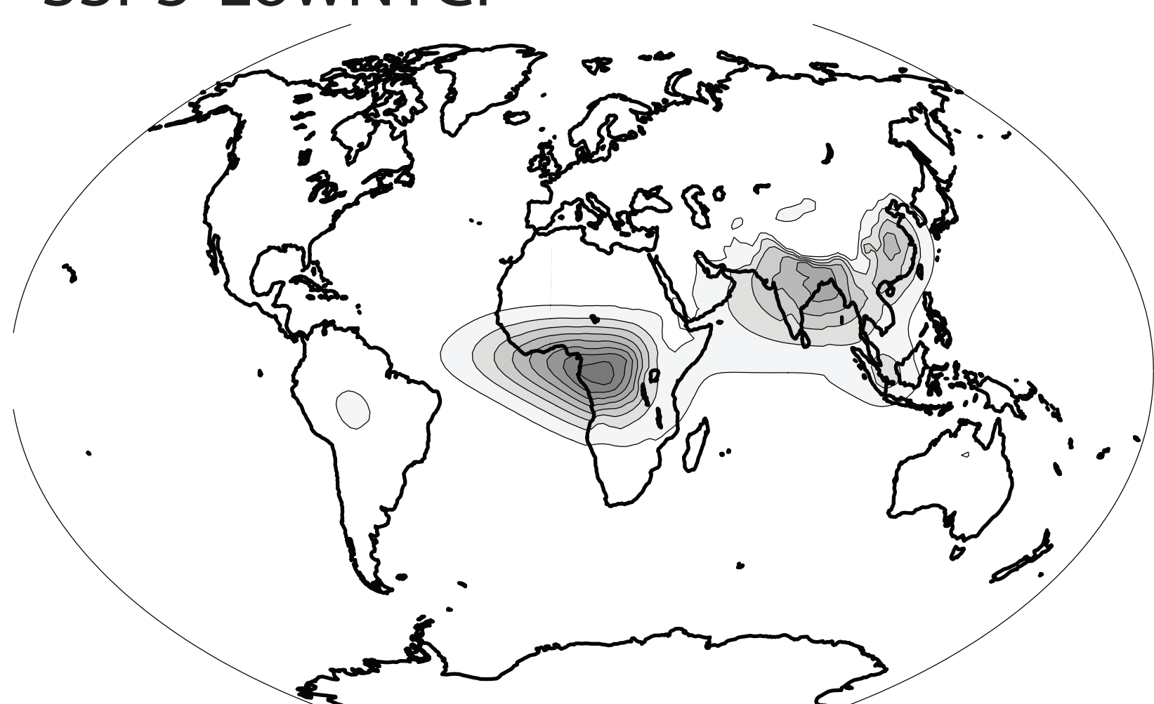
SSP3-LowNTCF
