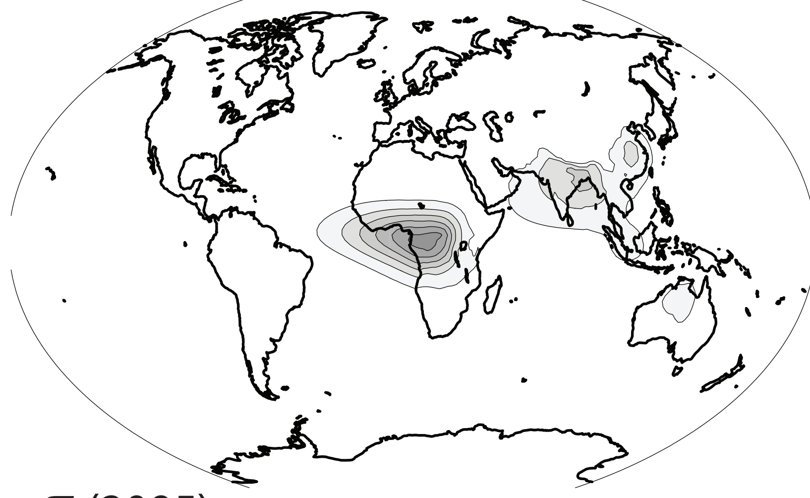
SSP5-34-OS
