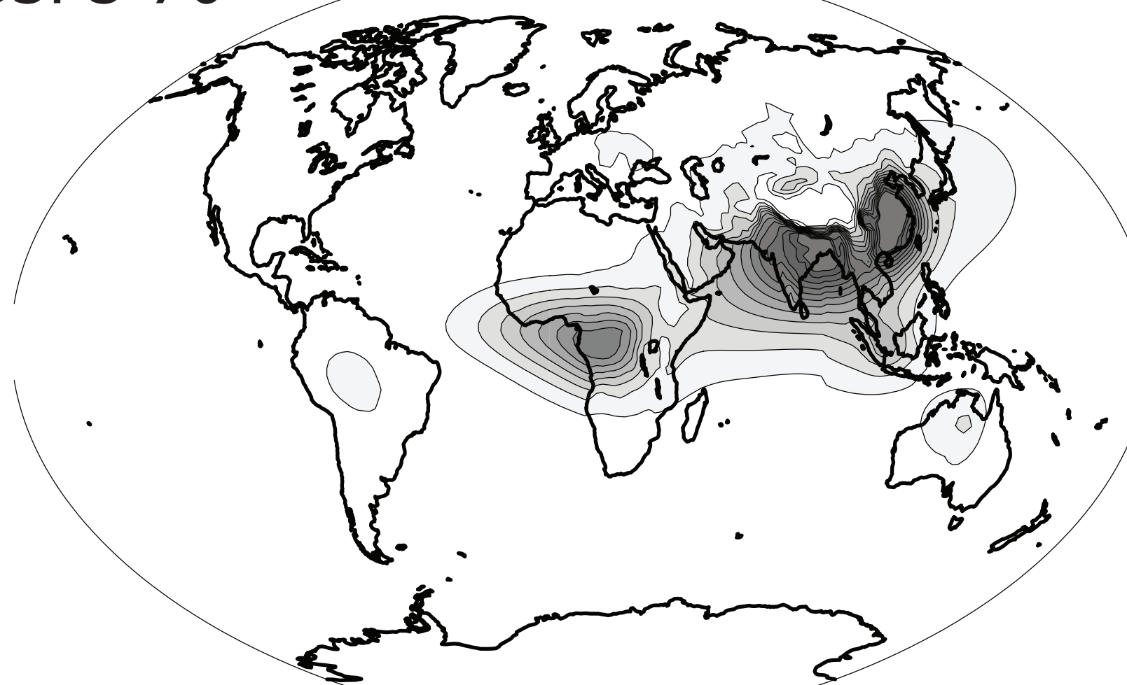
SSP3-70
