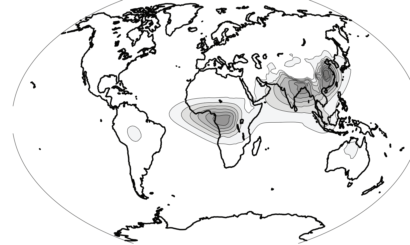
SSP3-LowNTCF
