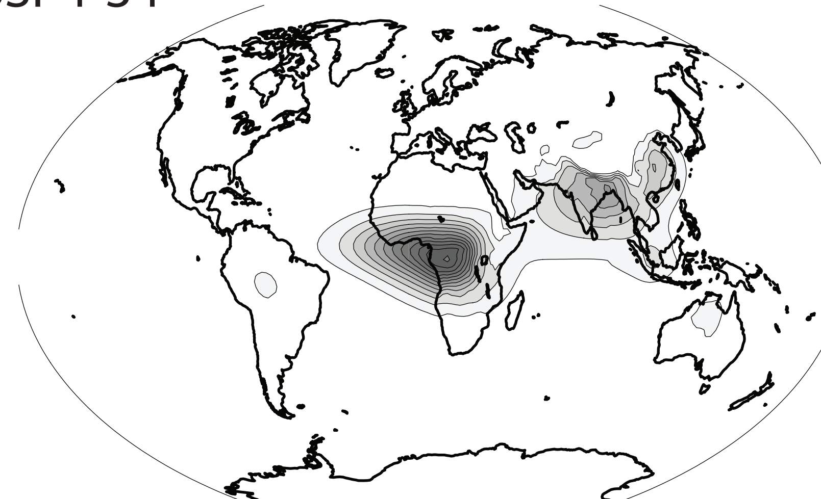
SSP4-34
