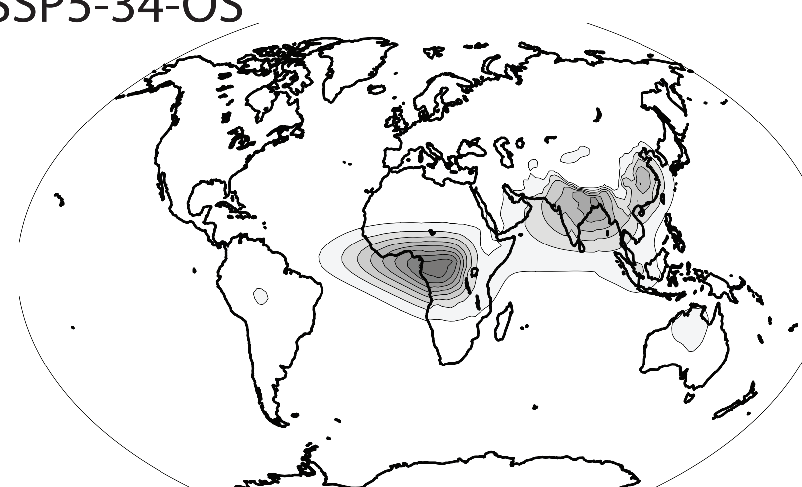
SSP5-85
