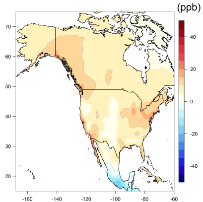
(b) GEOSCCM
