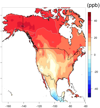
(e) MOCAGE
