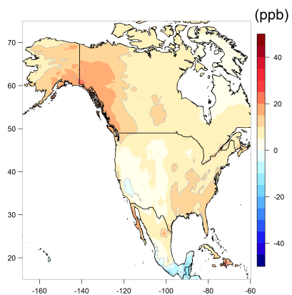
(d) G5NR-Chem
