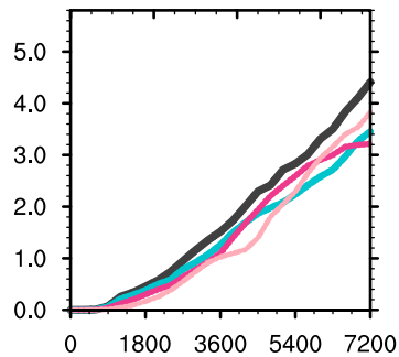
CSU
