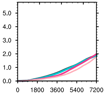
MPAS
