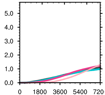
NICAM
