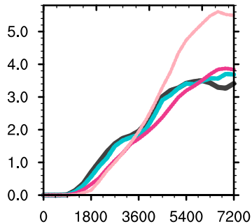
GEM
