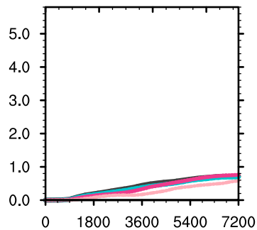
OLAM
