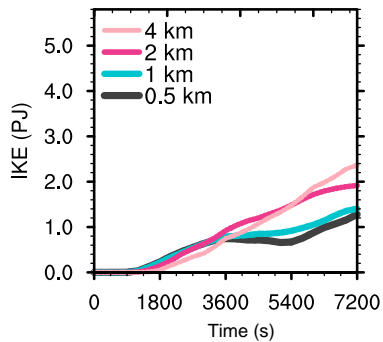
GEM
