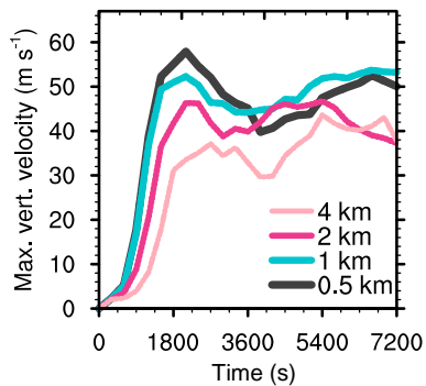
GEM
