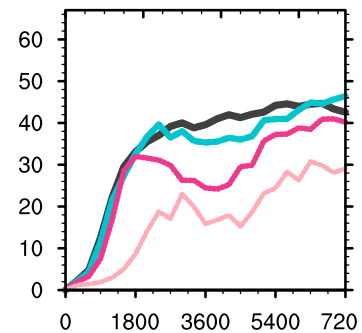
FVM
