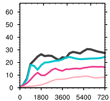
NICAM
