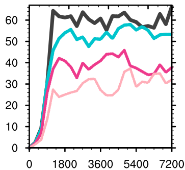
CSU
