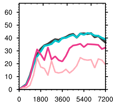
MPAS
