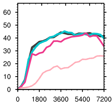
ICON
