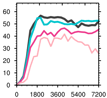
GEM
