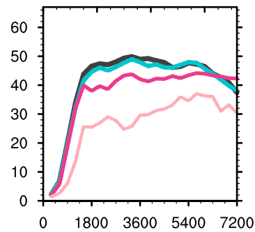
FV 3
