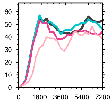
TEMPEST
