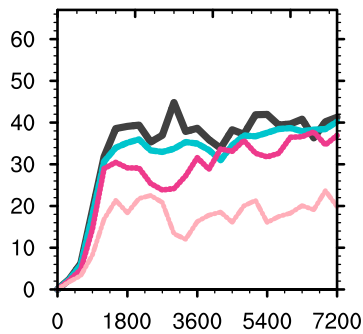
OLAM
