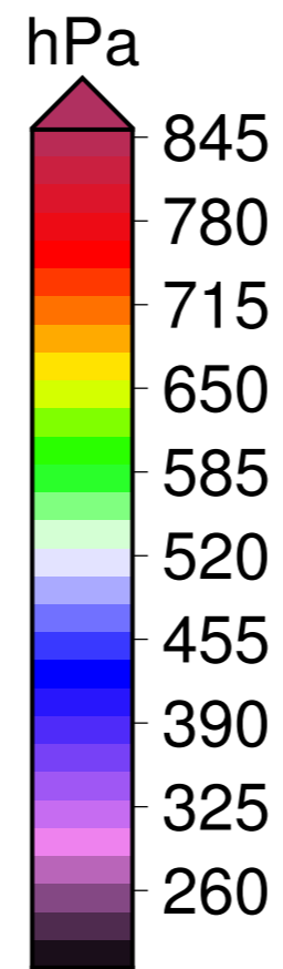
EC Earth - Cloud_cci
