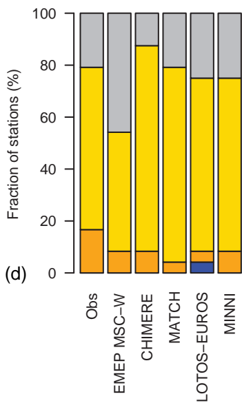
NO 2 1990-2000 (P1)
