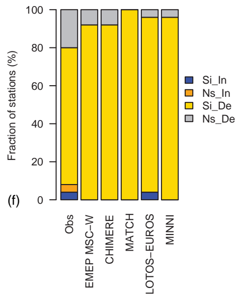
NO 2 1990-2010 (PT)
