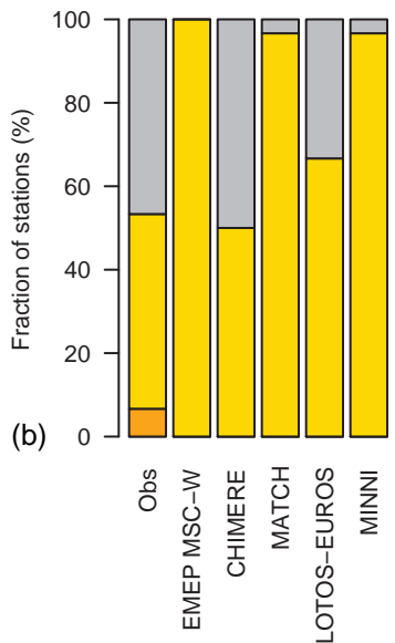
SO 2 2000-2010 (P2)
