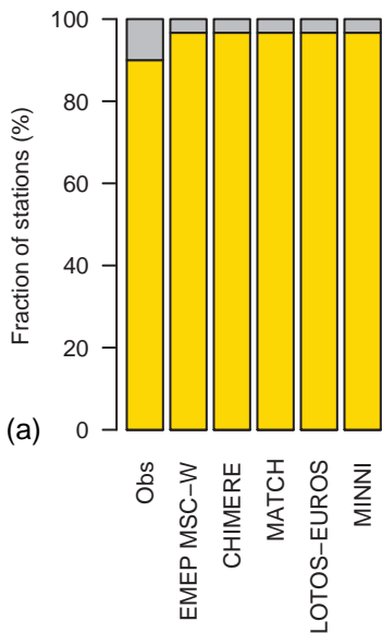
SO 2 1990-2000 (P1)
