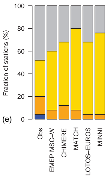
NO 2 2000-2010 (P2)
