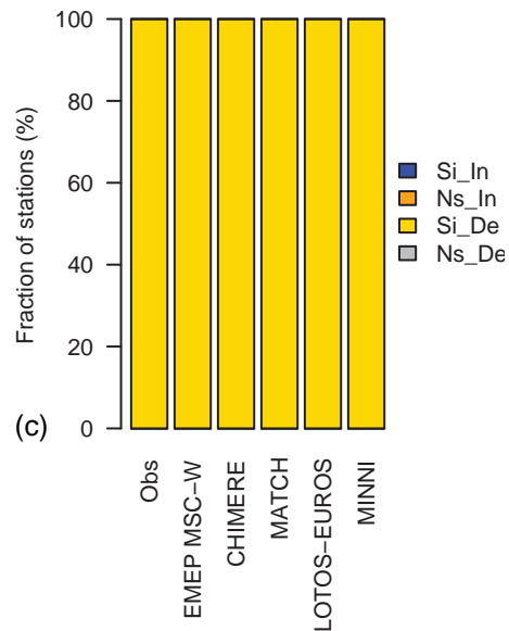
SO 2 1990-2010 (PT)
