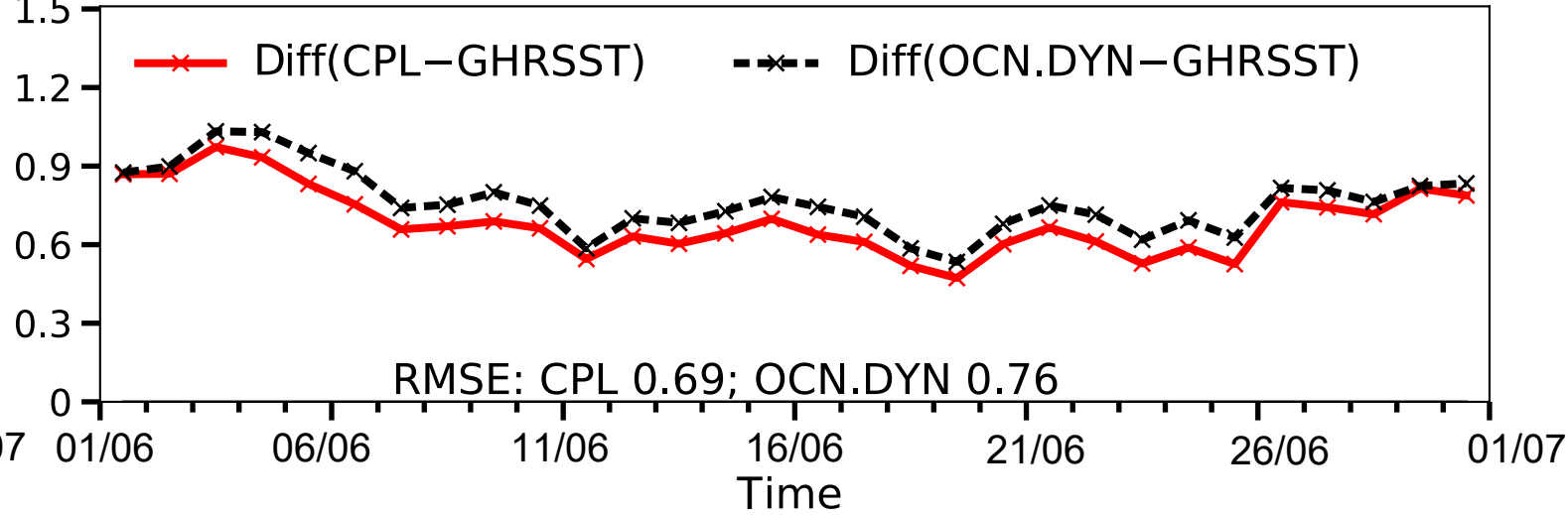
(b) Comparison with GHRSSST
