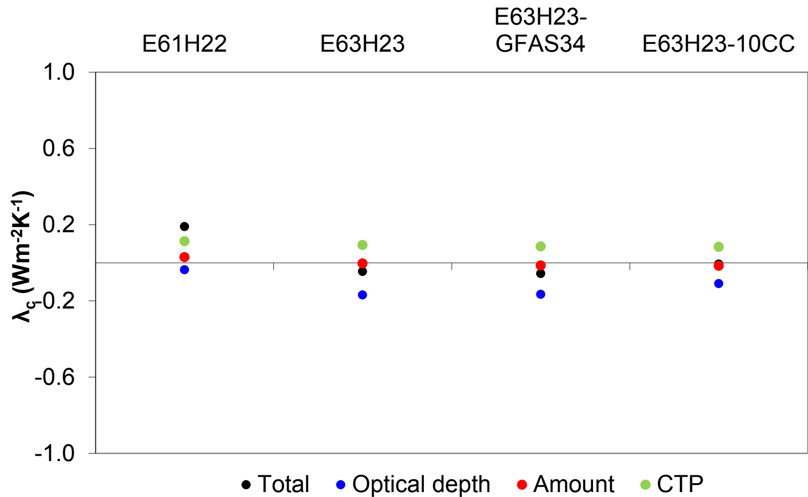
Net non-low cloud feedback parameter \lambda_c
