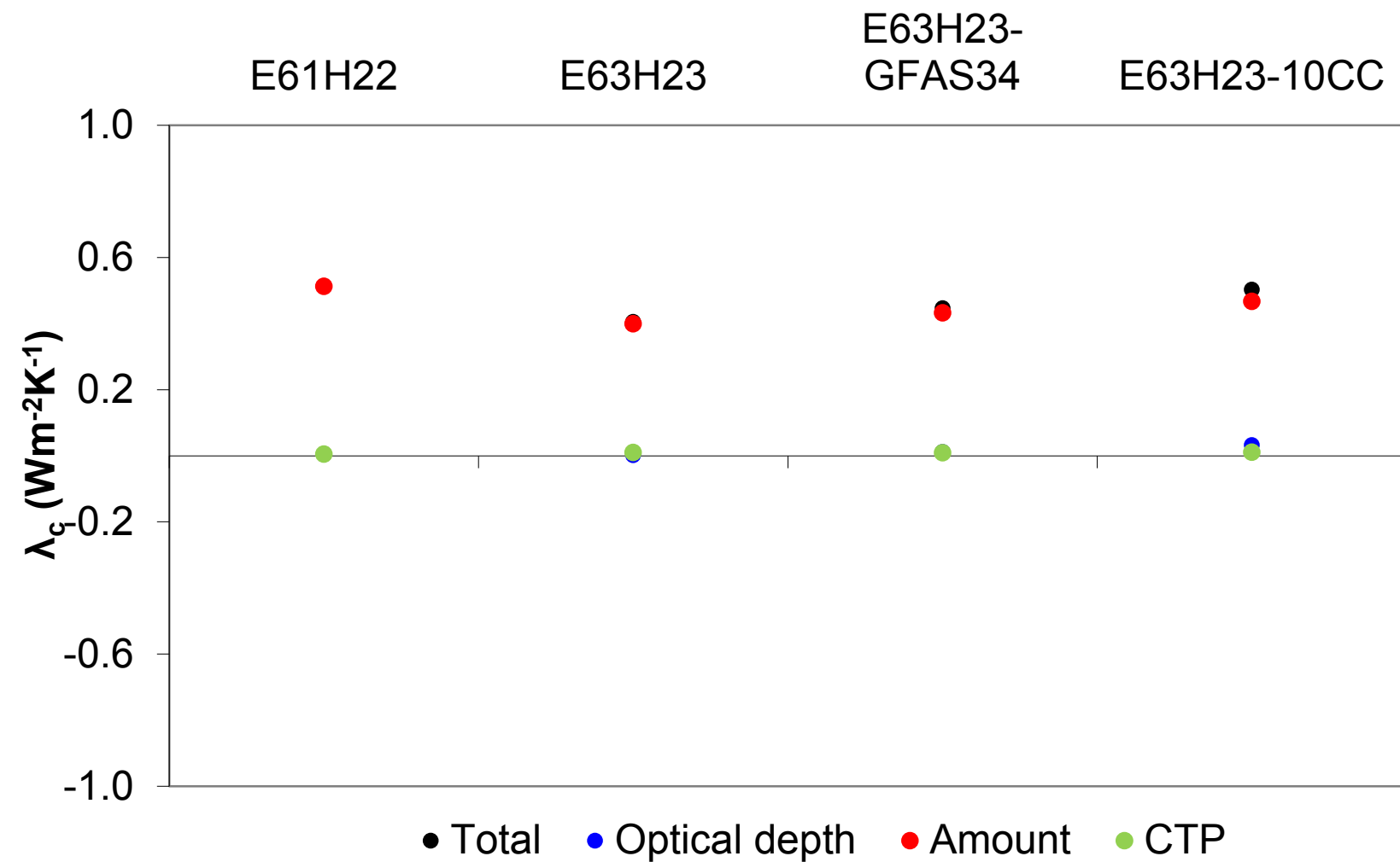
Net low cloud feedback parameter \lambda_c
