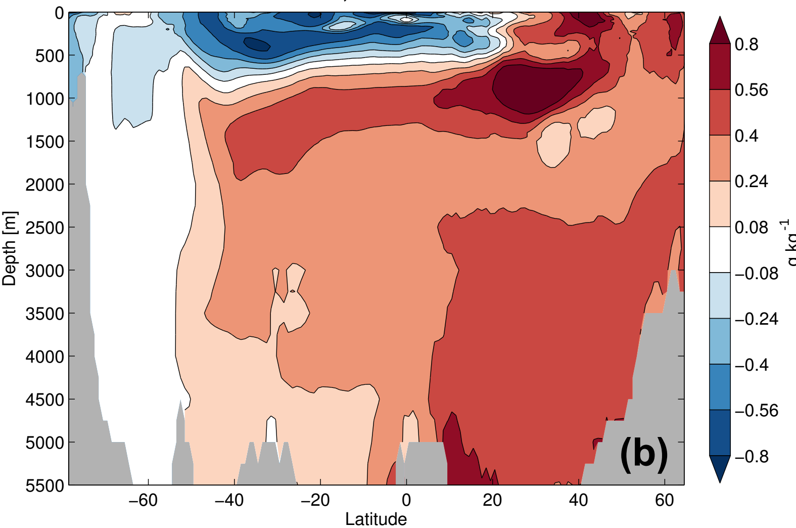
Atlantic zonal mean S, NorESM1-F minus WOA09
