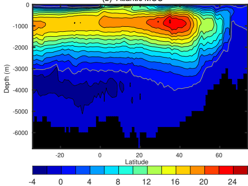
(b) Atlantic MOC
