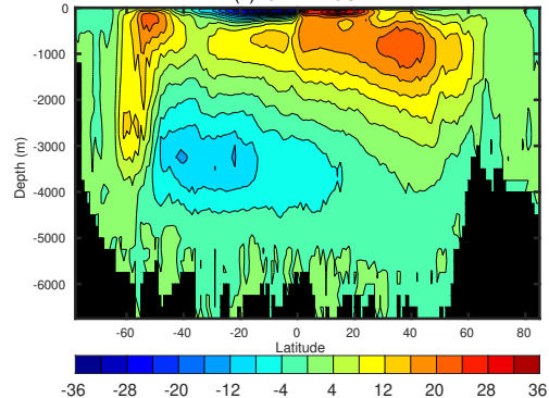
(a) Global MOC
