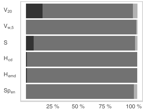
Observations : RS
