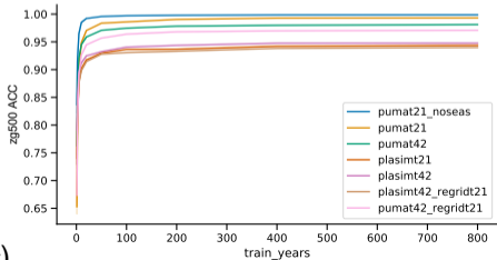
zg500 lead_time=1
