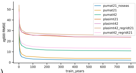
zg500 lead_time=1
