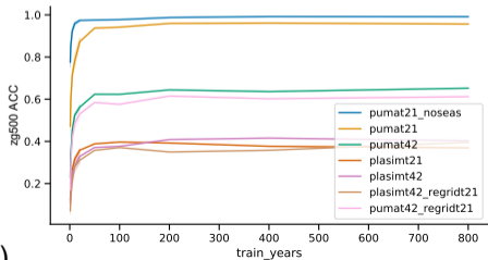
zg500 lead_time=6
