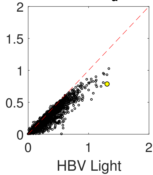
(d) KGE_a
