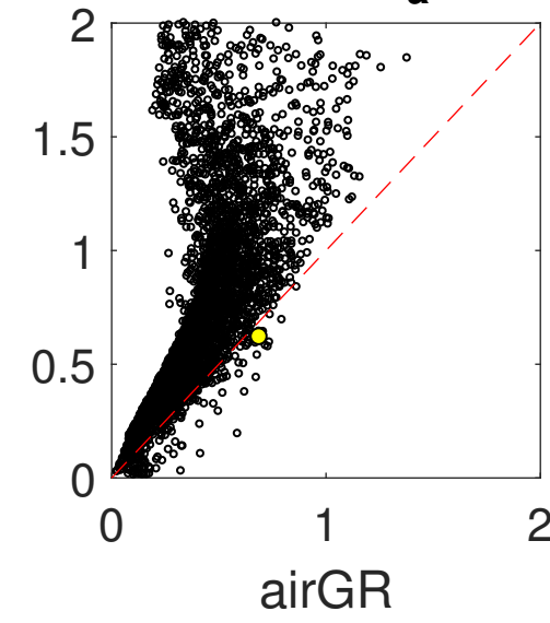
(g) KGE_a
