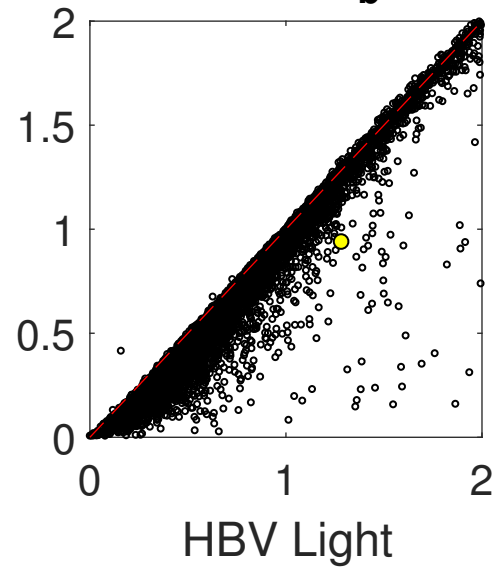
(e) KGE_b
