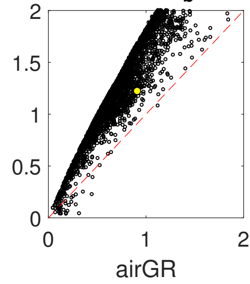
(h) KGE_b
