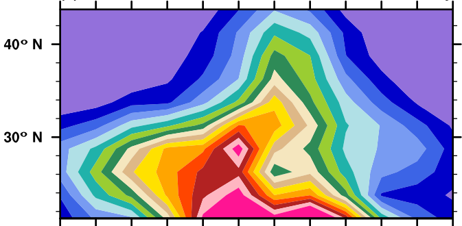
(a) GPCP
