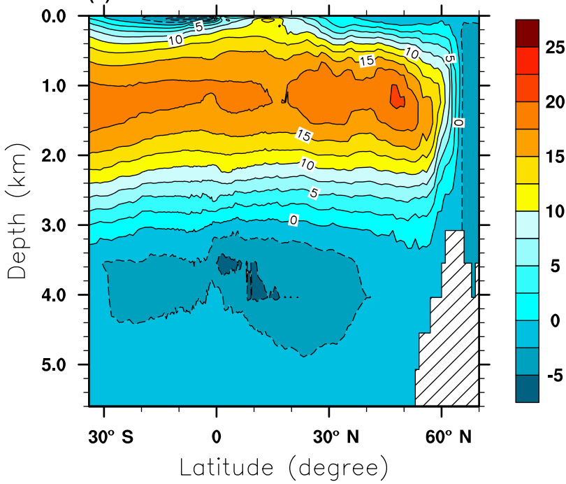
(b) BCC-CSM1.1m
