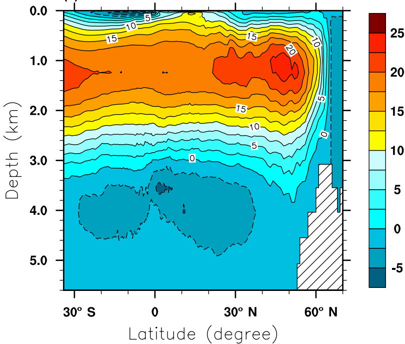
(b) BCC-CSM1.1m
