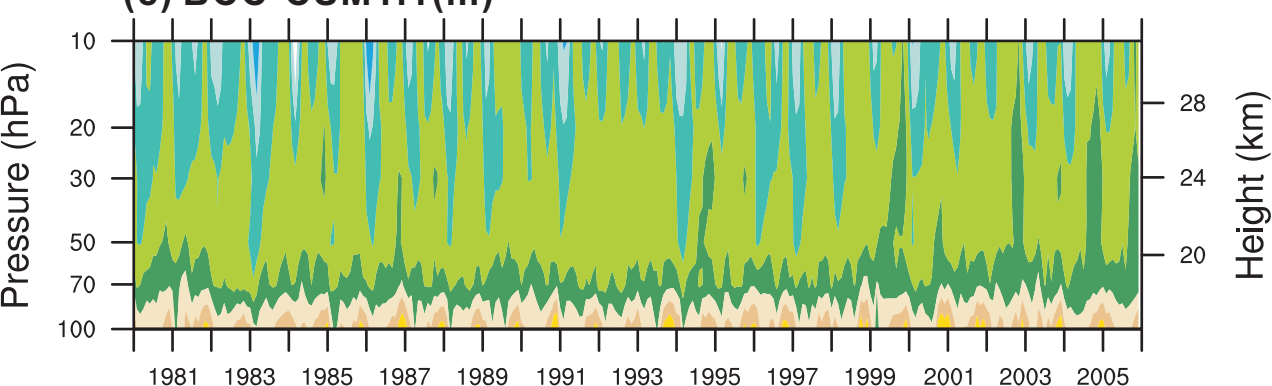
(c) BCC-CSM1.1(m)
