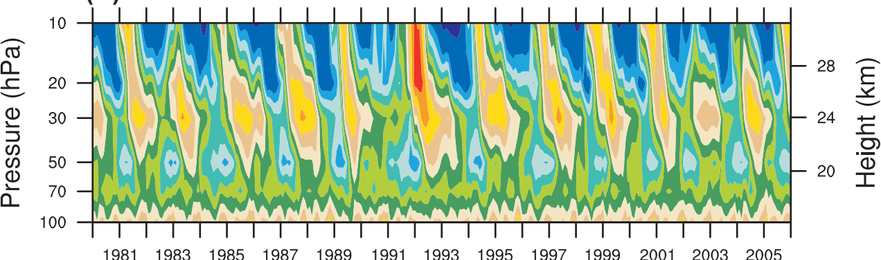
(c) BCC-CSM1.1(m)
