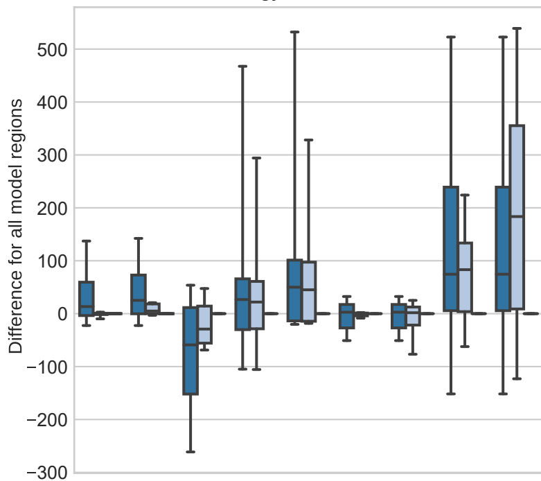
Energy sector CO2
