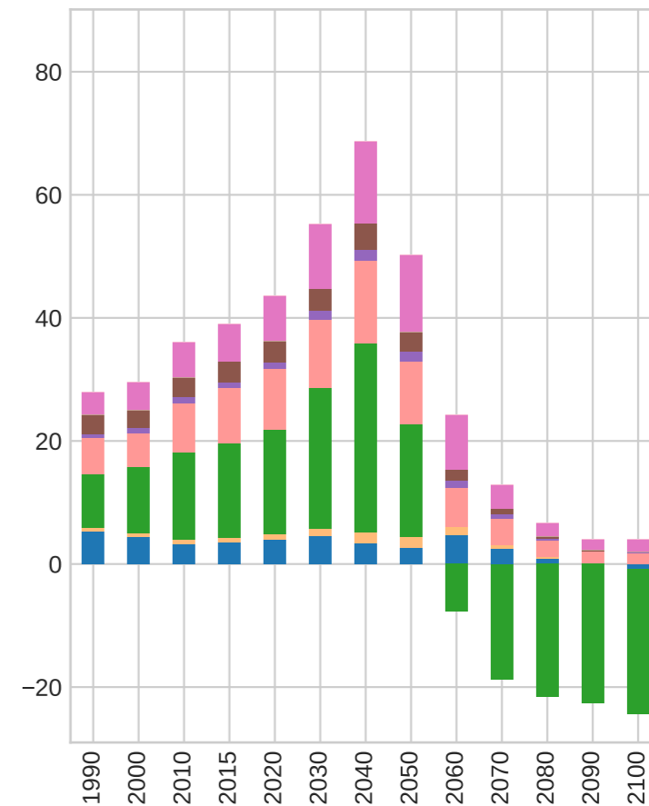
SSP5-3.4-OS CO2
