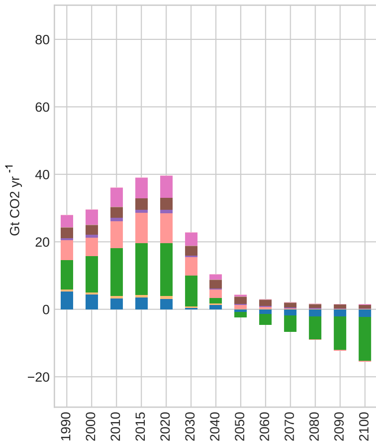
SSP1-1.9 CO2
