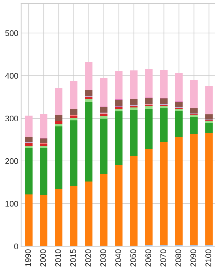
SSP4-3.4 CH4
