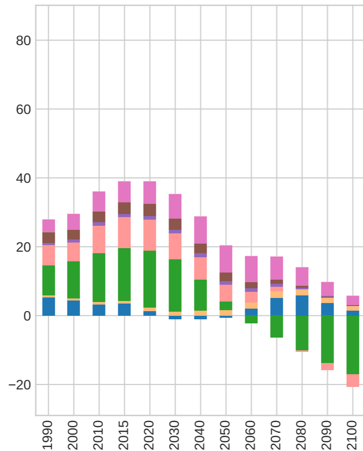
SSP4-3.4 CO2
