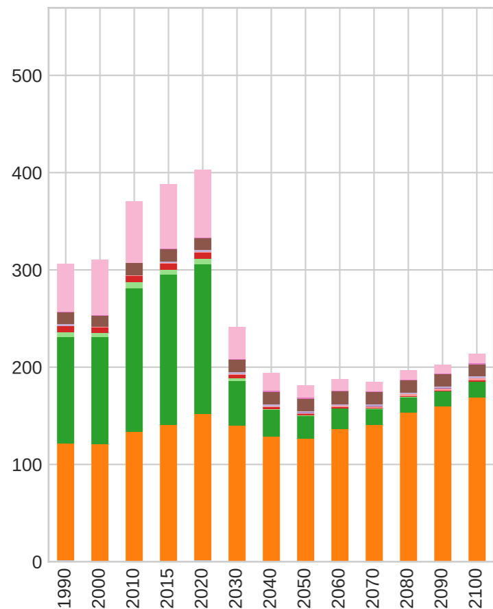
SSP3-LowNTCF CH4
