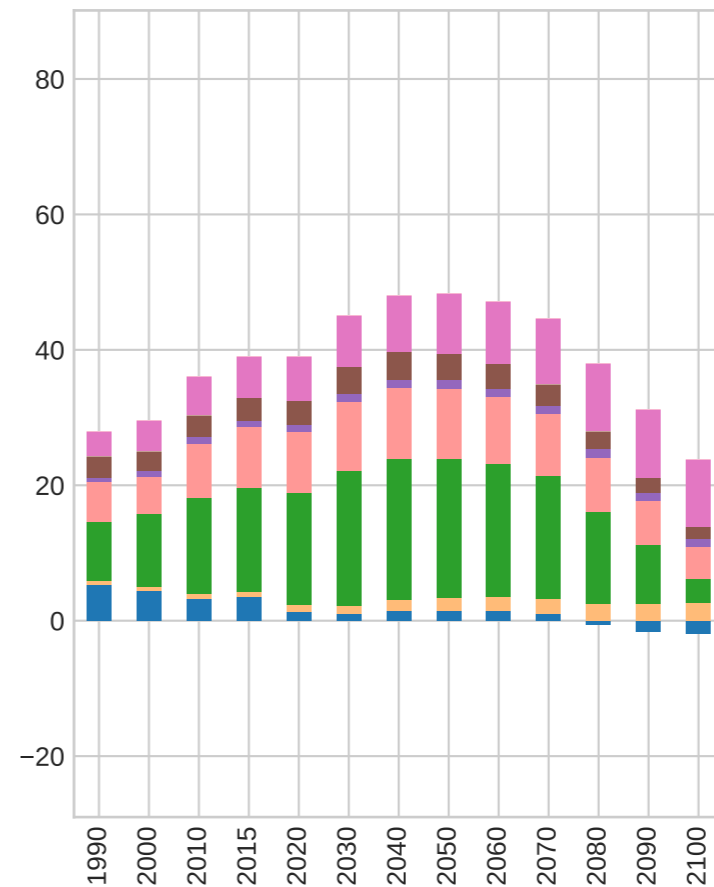
SSP4-6.0 CO2
