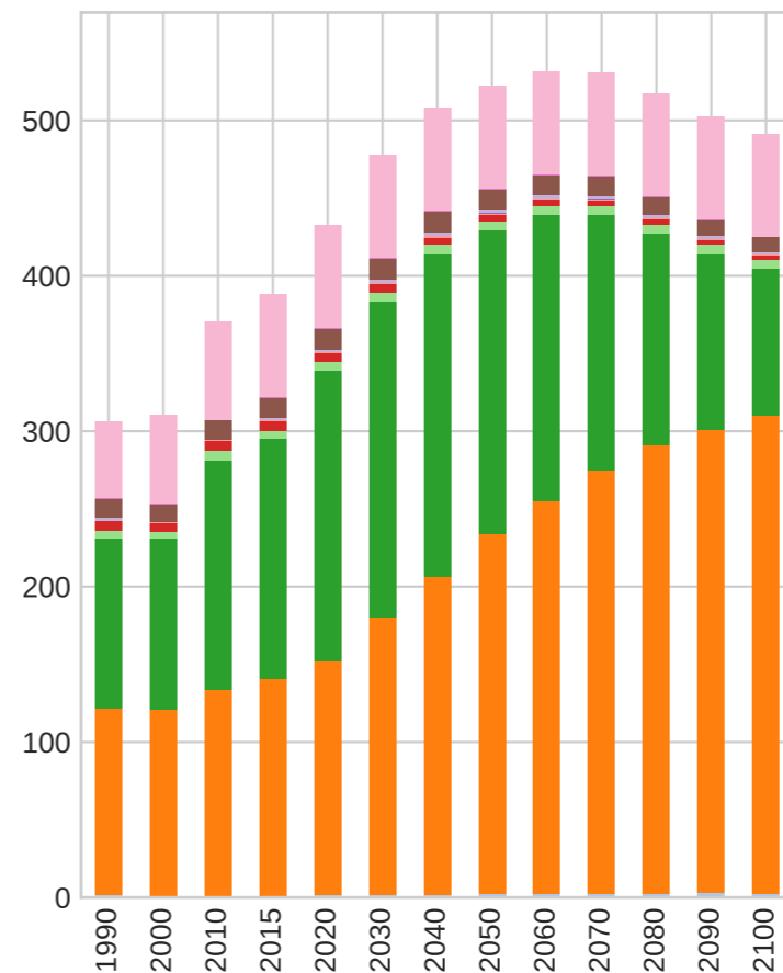
SSP4-6.0 CH4
