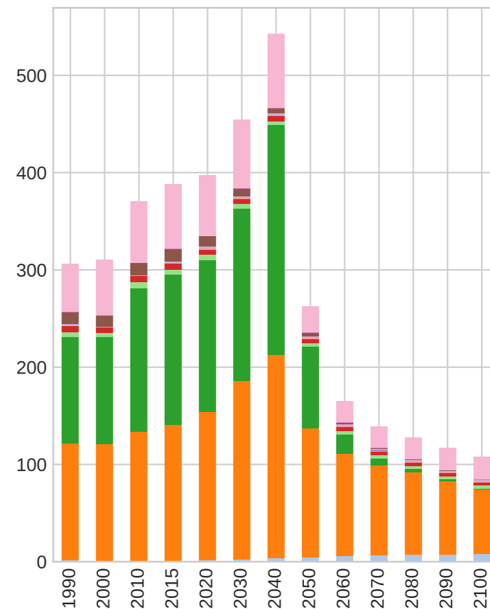
SSP5-3.4-OS CH4
