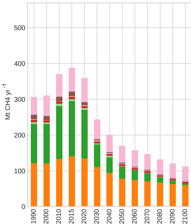
SSP1-1.9 CH4
