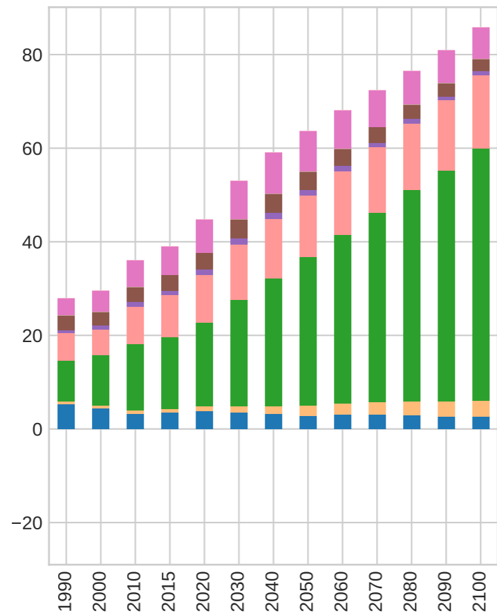
SSP3-LowNTCF CO2
