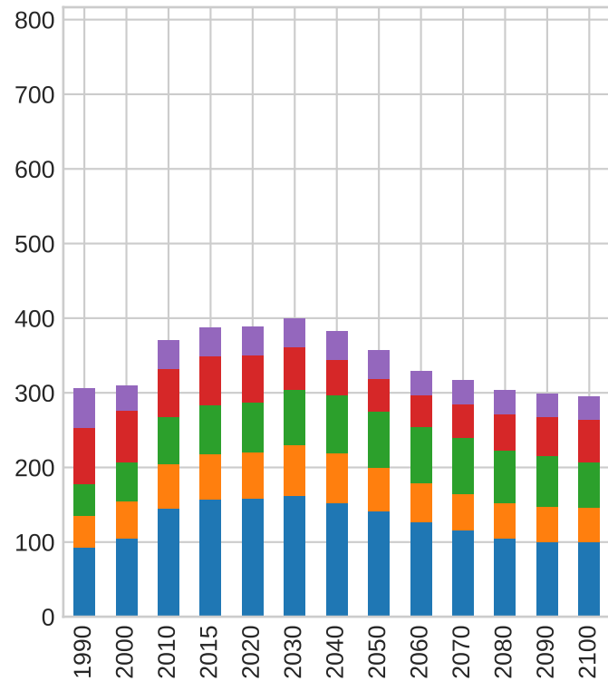
SSP2-4.5 CH4
