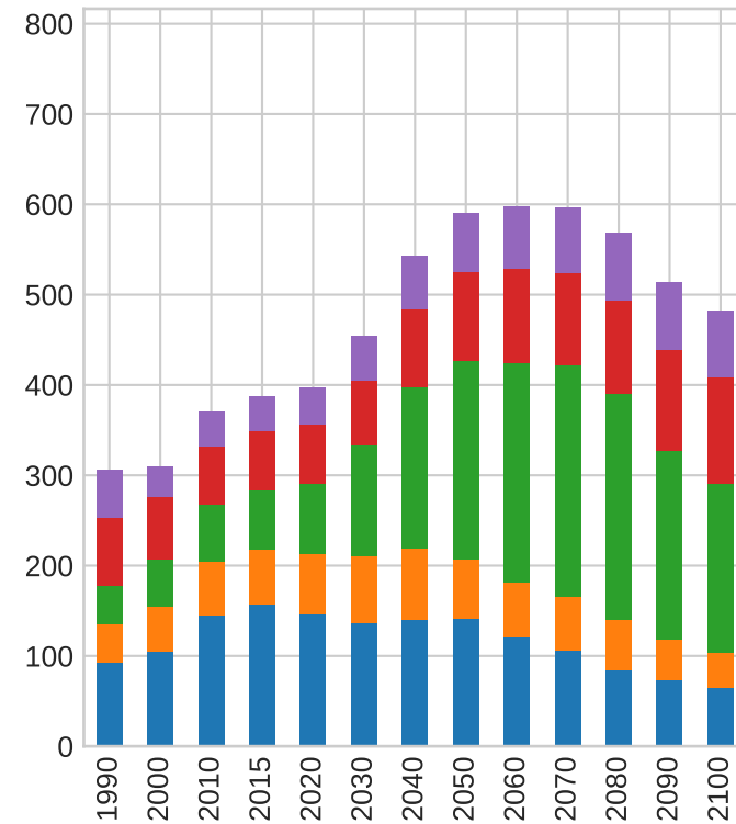
SSP5-8.5 CH4
