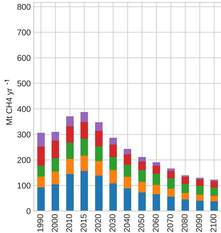
SSP1-2.6 CH4
