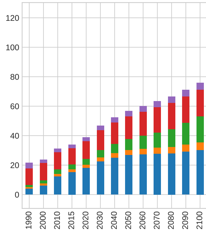
SSP3-7.0 CH4
