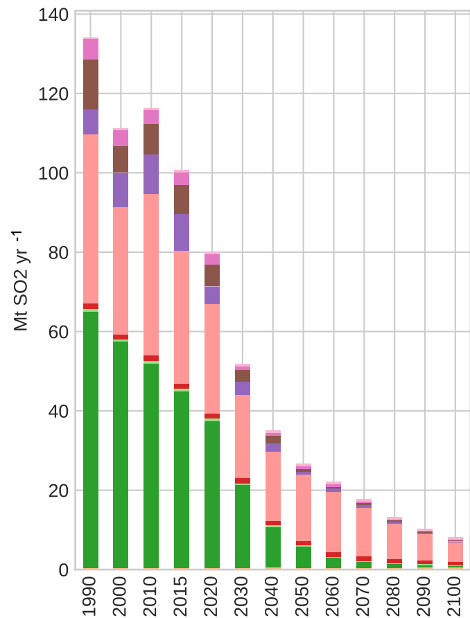
SSP1-2.6 sulfur
