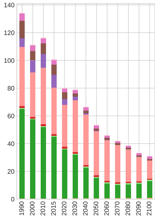
SSP2-4.5 sulfur
