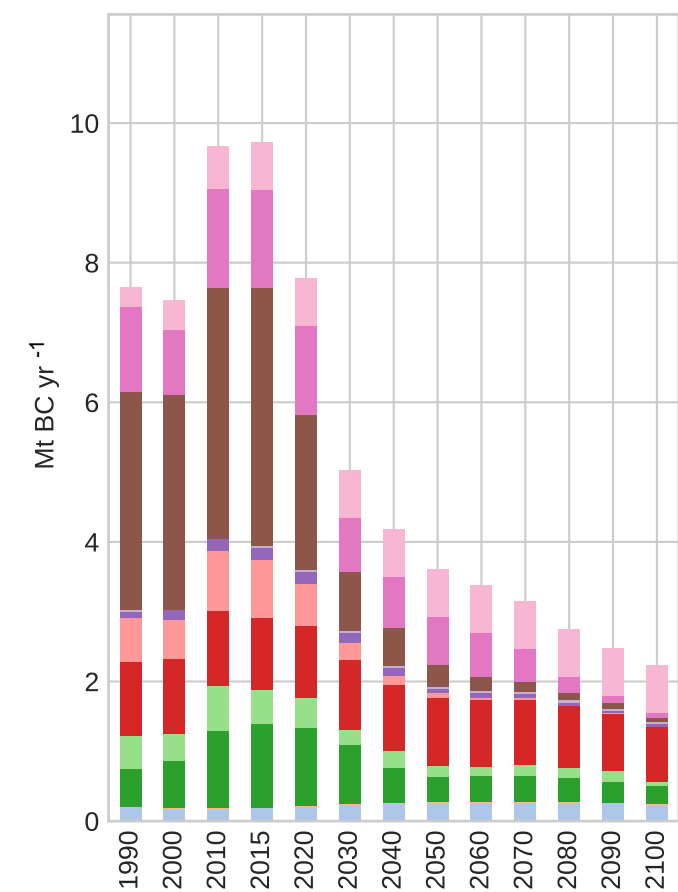
SSP1-2.6 BC
