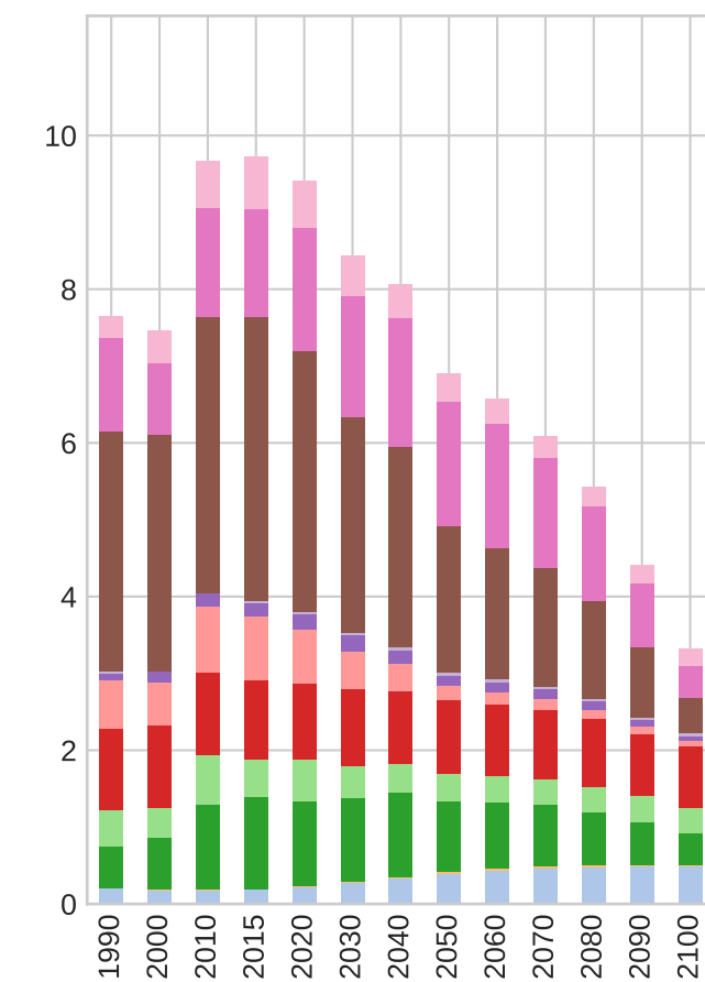
SSP5-8.5 BC
