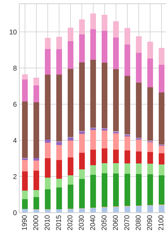
SSP3-7.0 BC
