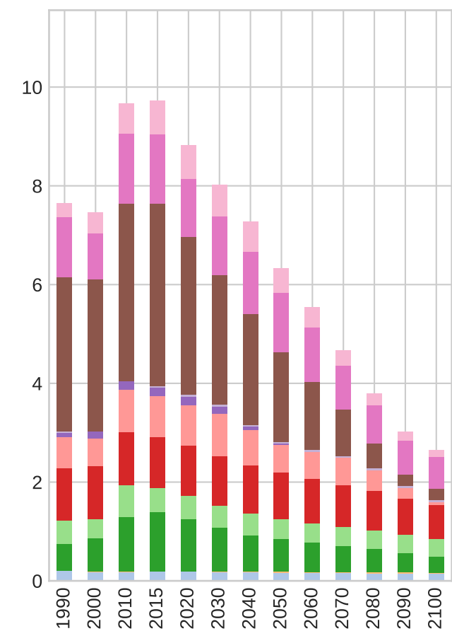
SSP2-4.5 BC
