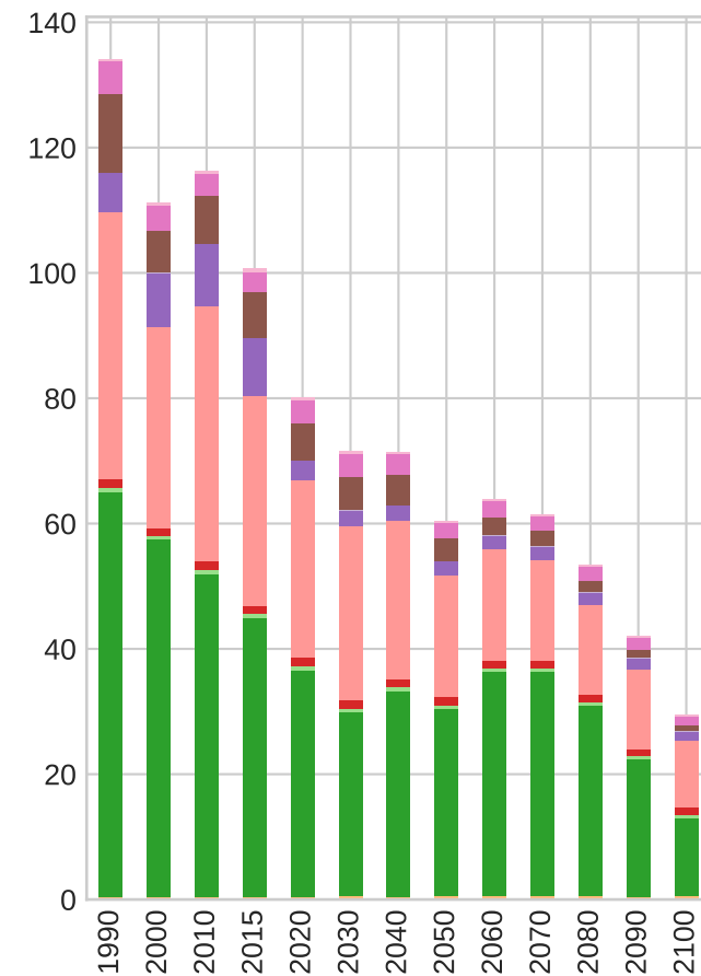
SSP5-8.5 sulfur
