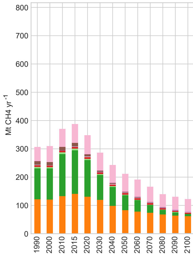
SSP1-2.6 CH4
