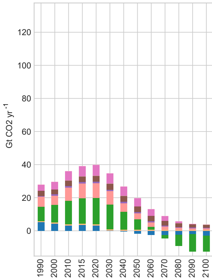
SSP1-2.6 CO2
