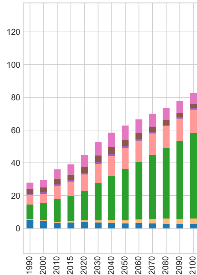
SSP3-7.0 CO2
