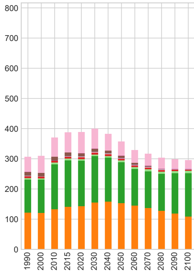
SSP2-4.5 CH4
