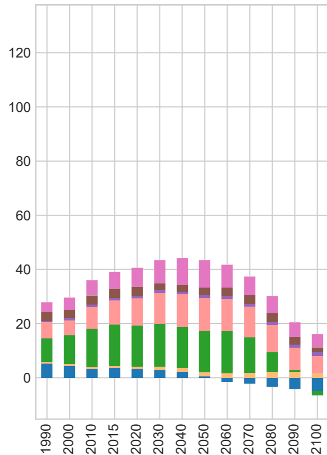
SSP2-4.5 CO2
