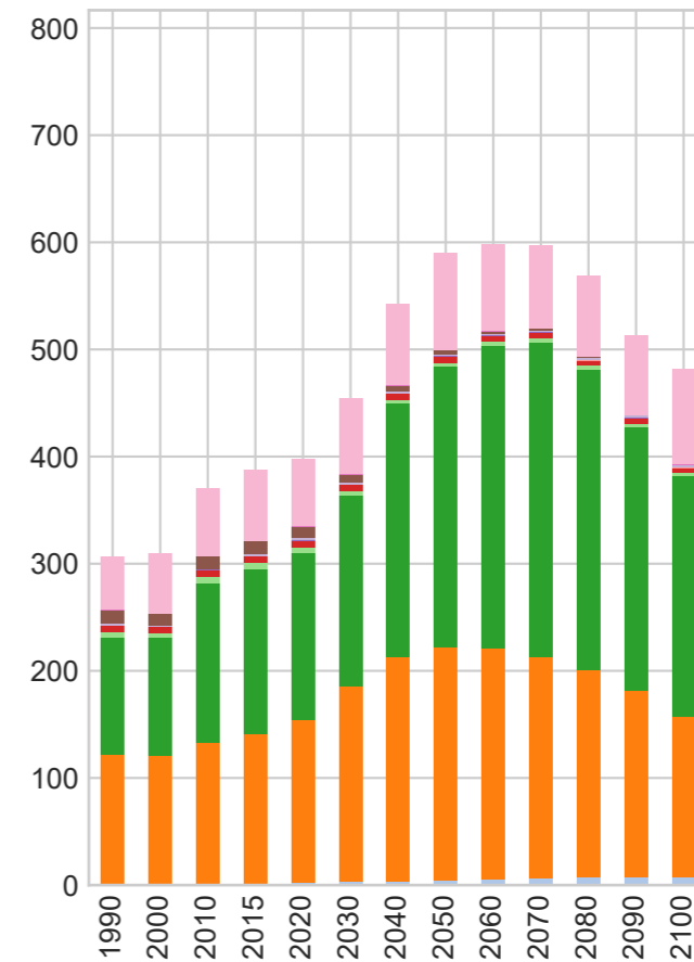
SSP5-8.5 CH4
