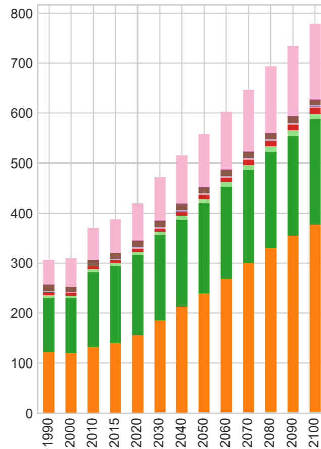
SSP3-7.0 CH4
