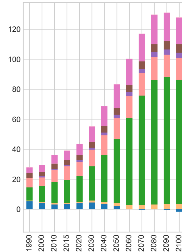
SSP5-8.5 CO2
