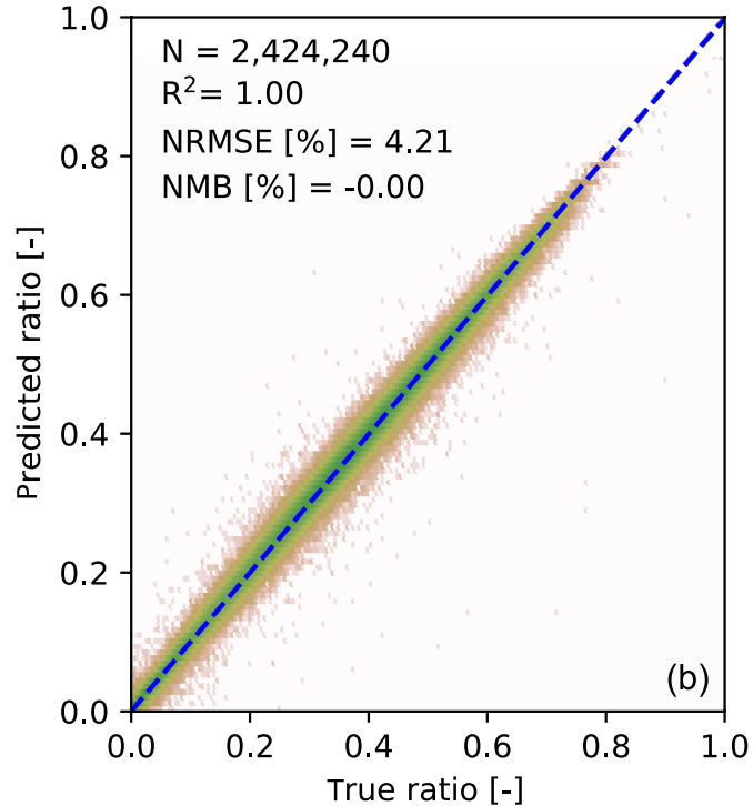
NO:NOx ratio
