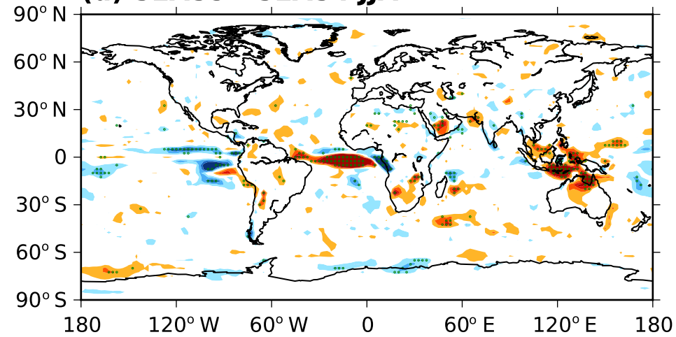
(d) SEAS5 - SEAS4 JJA
