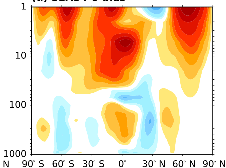
(d) SEAS4 U bias
