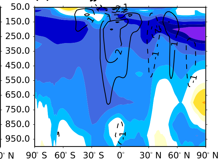
(d) SEAS4 JJA bias
