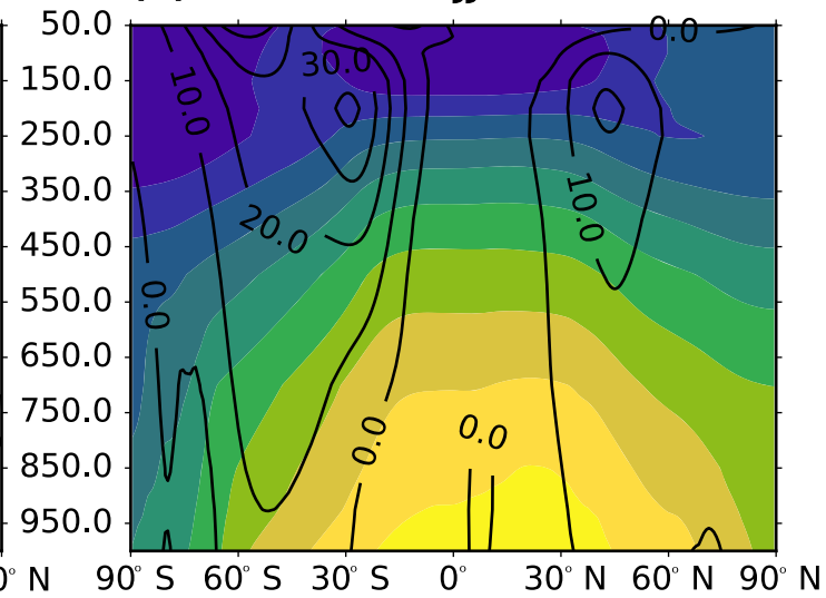
(b) ERA-Interim JJA
