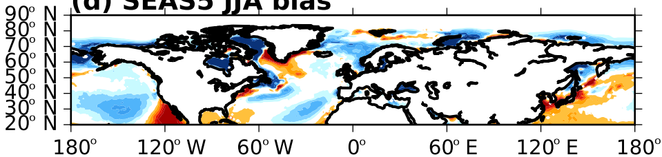
(d) SEAS5 JJA bias
