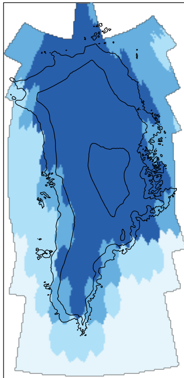
(b) ISCCP
