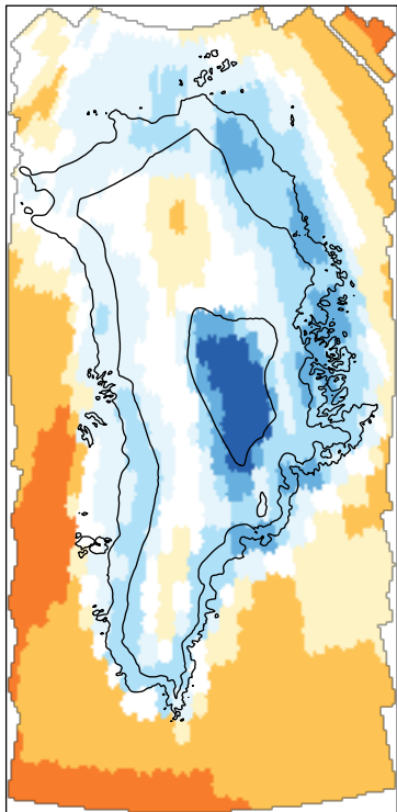
(a) CESM
