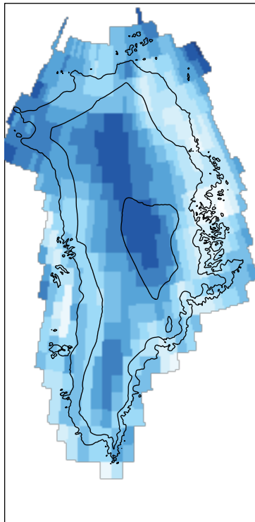
(a) CESM, LW_{net}
