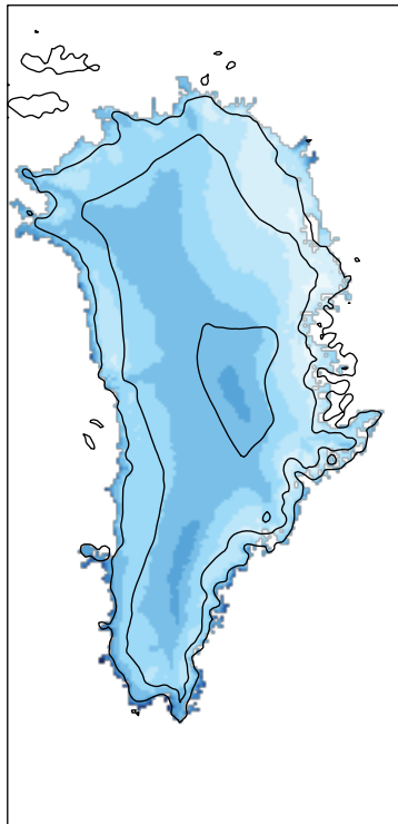
(b) RACMO, LW_{net}
