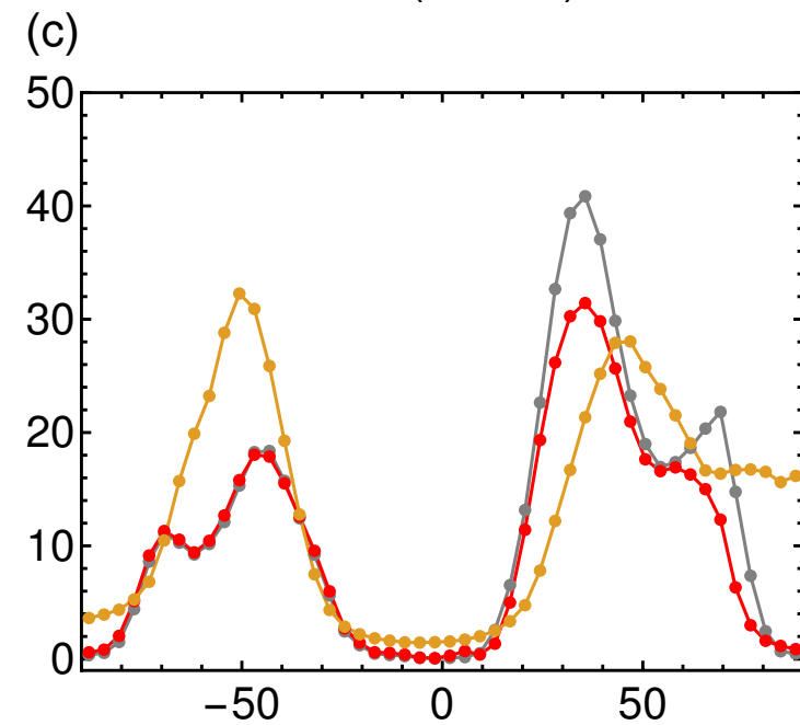
La Niña (500 mb)
