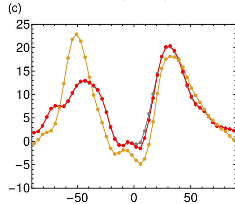
La Niña (500 mb)
