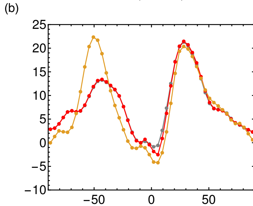
El Niño (500 mb)
