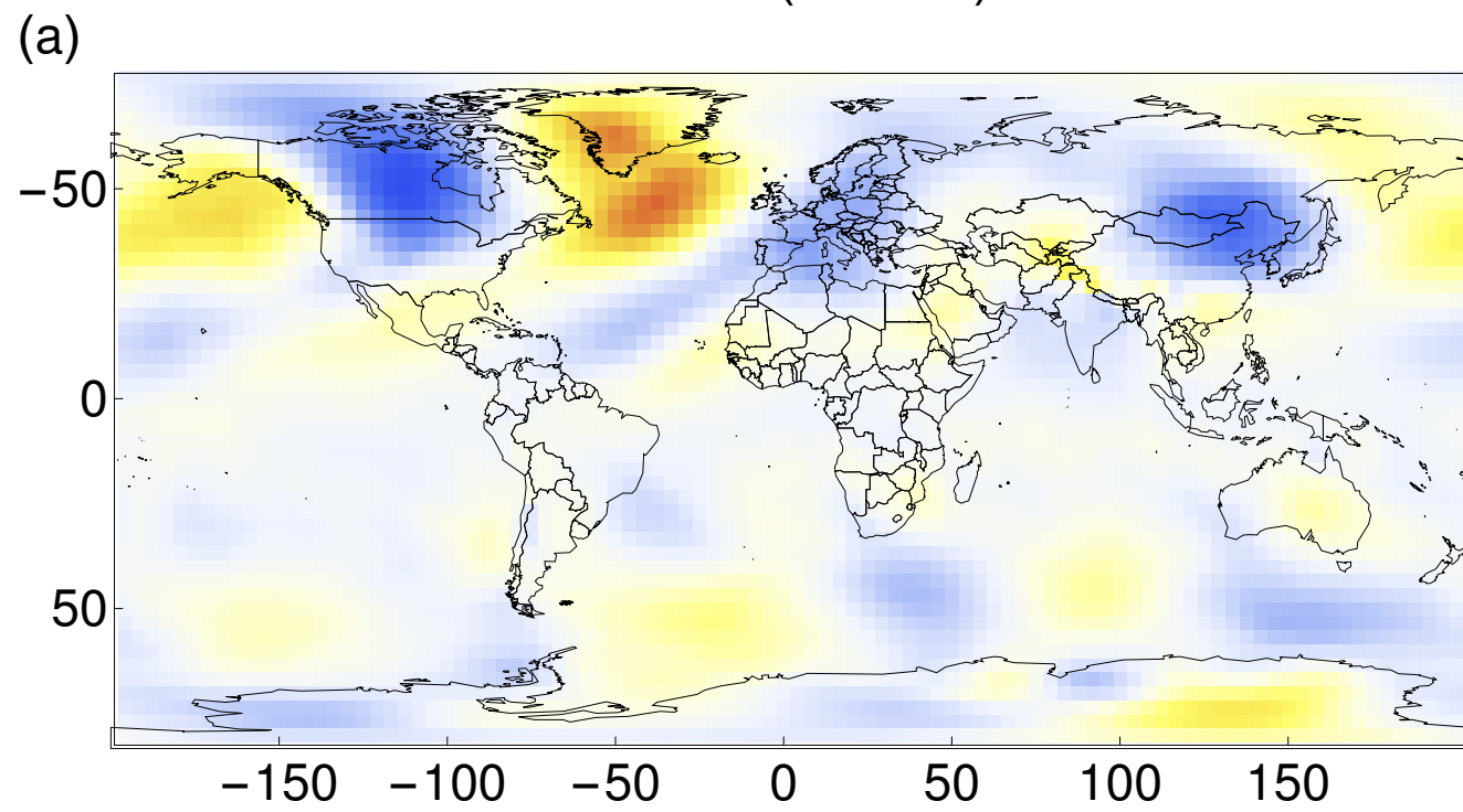
ERA-Interim v^* (500 mb)
