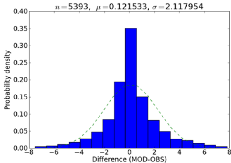
(b) CTEM-GEM
