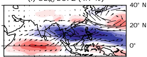
(f) GL 90 EOF2 (4.7 %)
