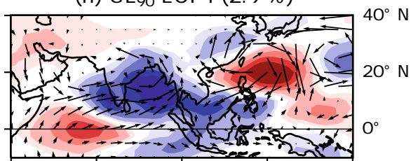
(h) GL 90 EOF4 (2.9 %)
