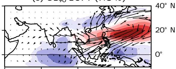
(e) GL 90 EOF1 (7.8 %)
