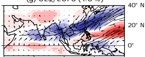
(g) GL 90 EOF3 (4.3 %)
