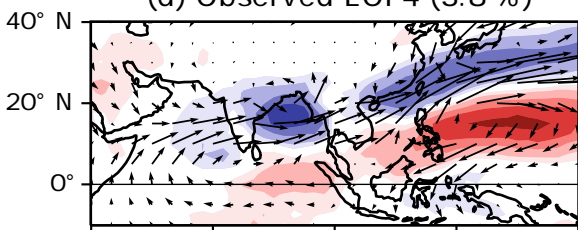
(d) Observed EOF4 (3.8 %)
