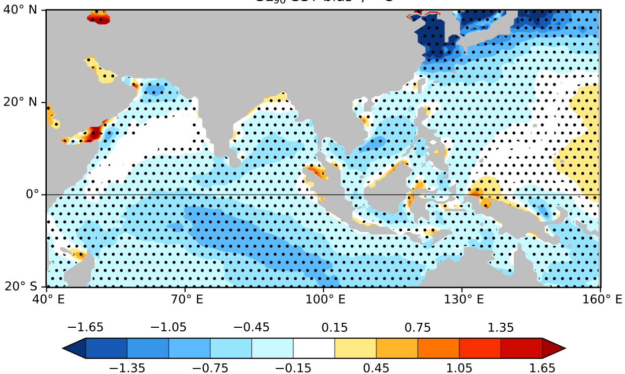
GL 90 SST bias / °C
