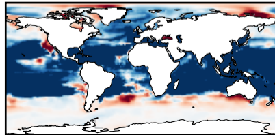
(d) Quotient
