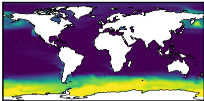
(a) HadGEM2-ES
