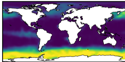
(b) WOA
